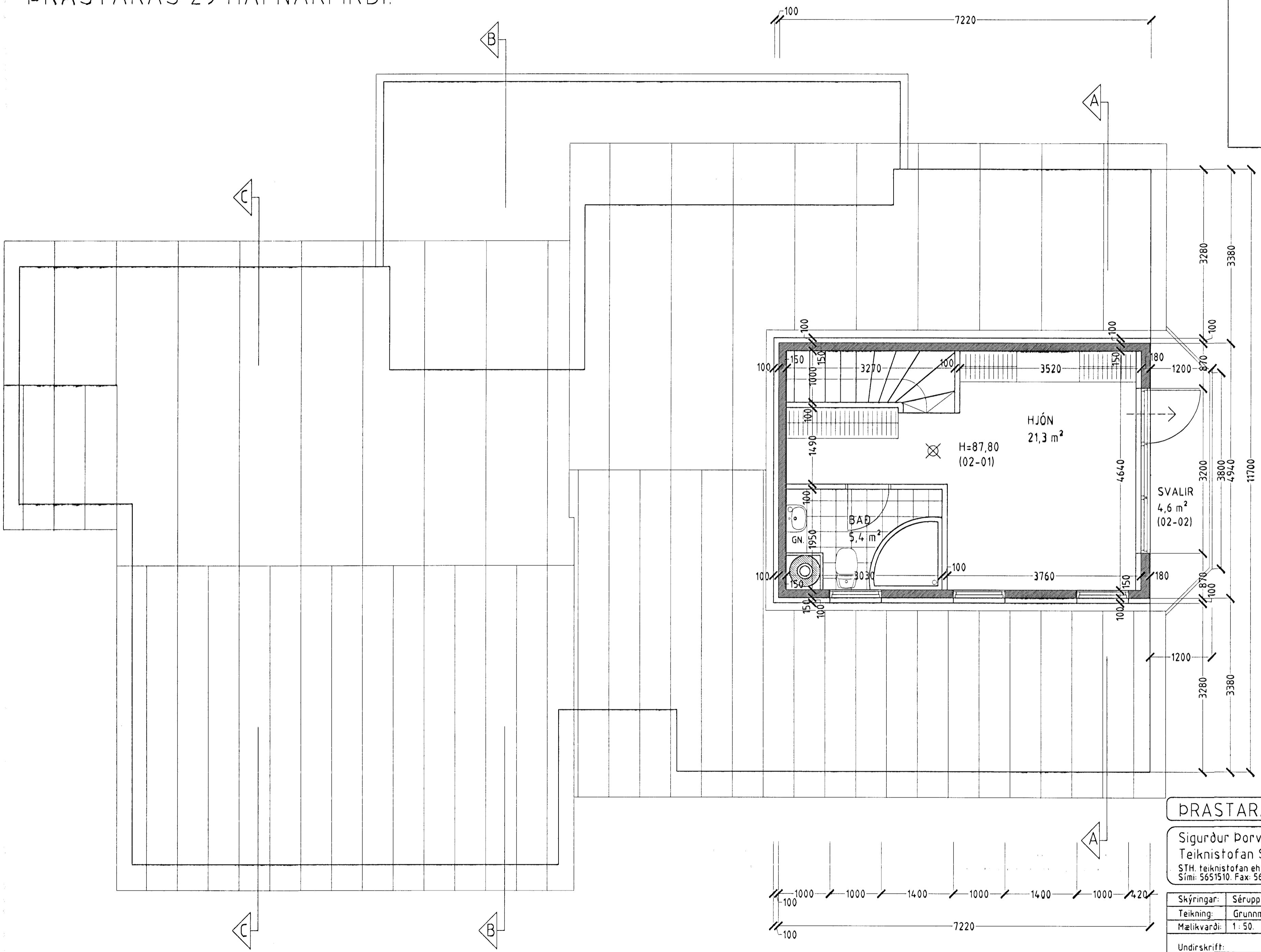
GRUNNMYND 2 HÆÐ MKV. 1:50.
