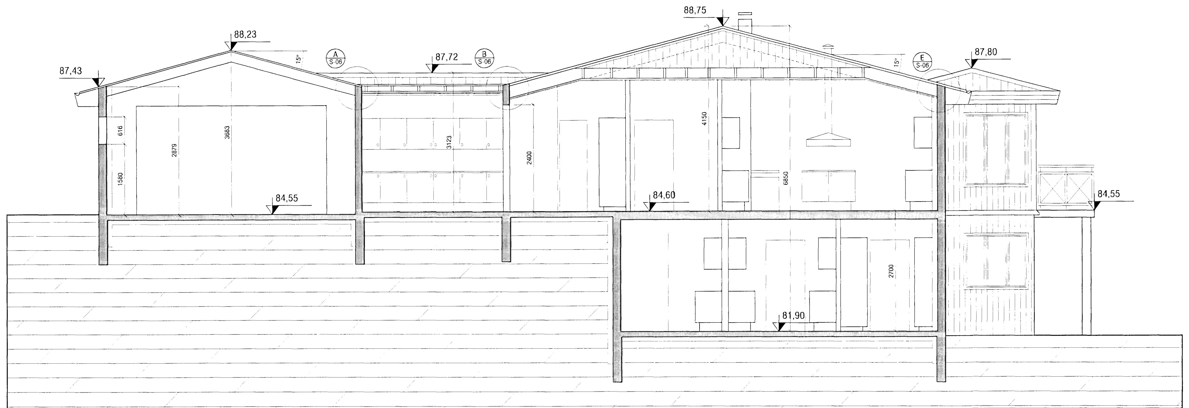
SNID A-A
