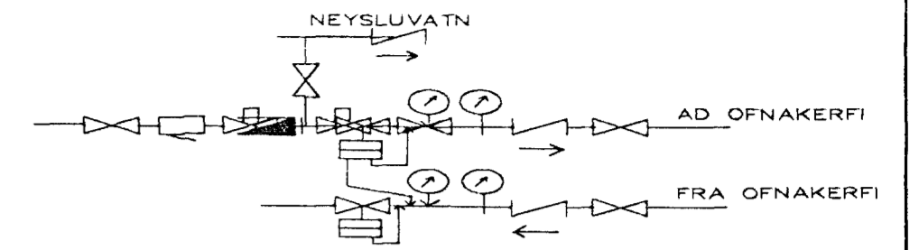
MÆLAGRIND HITAVEITU
