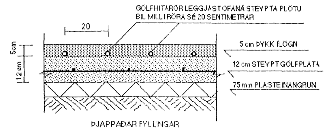
SNID Í STEYPTA PLÖTU MEÐ GÖLFHITA MKY. 1:10
