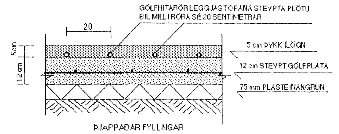
SNID I STEYPTA PLÖTU MED GÓLFHITA MKY. 1:10
