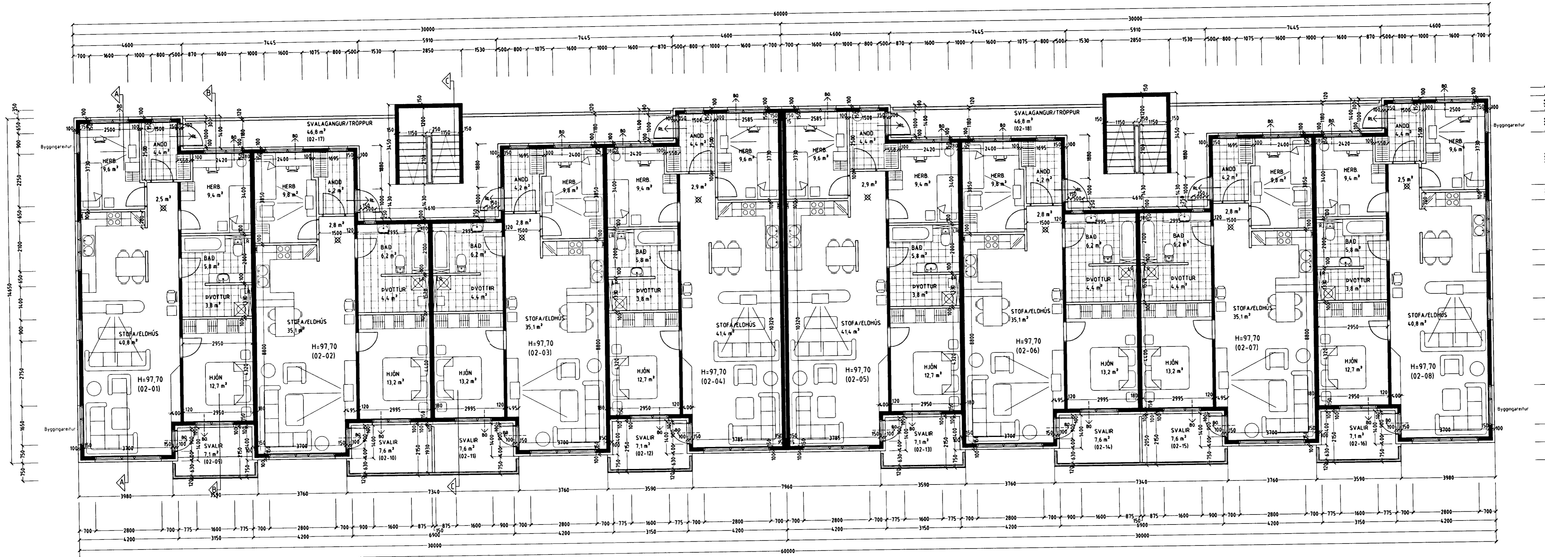
GRUNNMYND 2 HÆÐ. MKV. 1:100.
