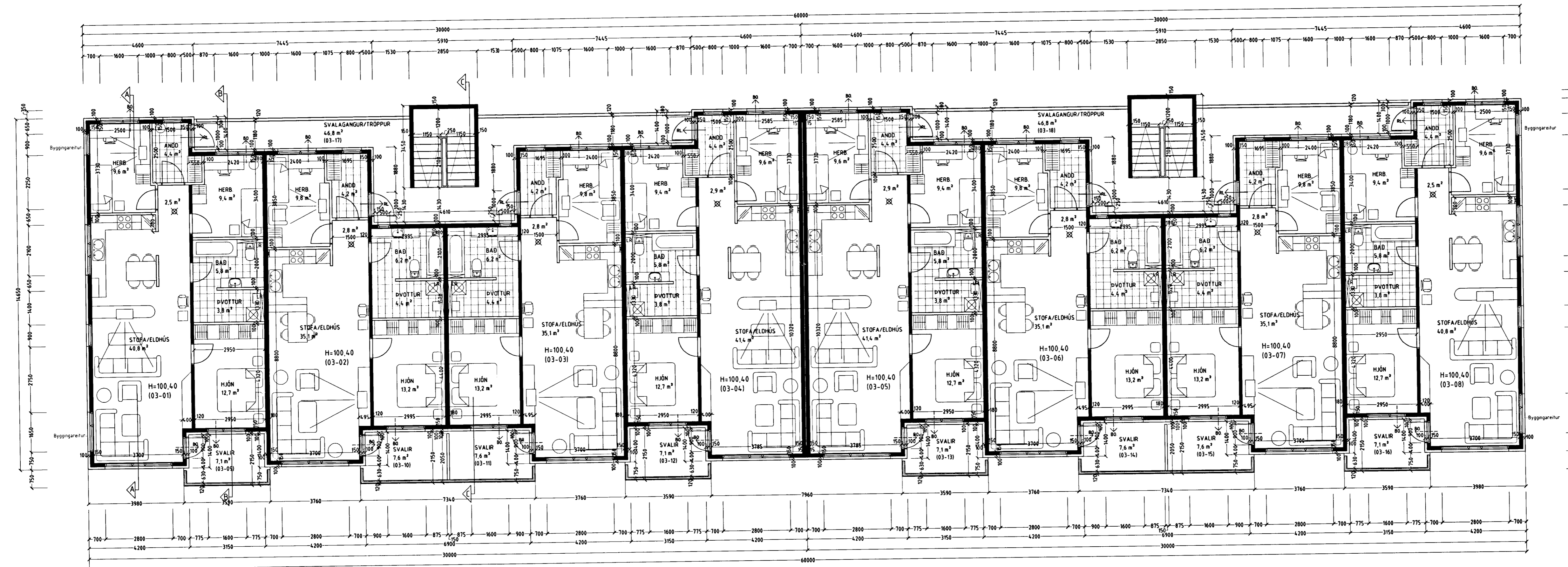
GRUNNMYND 3 HÆÐ. MKV. 1:100.
