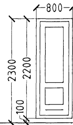
2 STK STÓFA & HJÓN HURÐ OP ÚT V.
