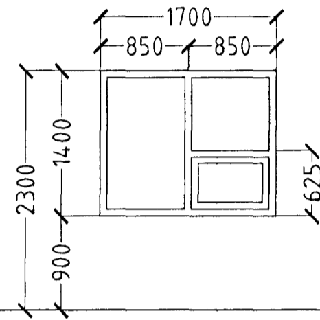
4 STK HERB. & ELDHÚS
