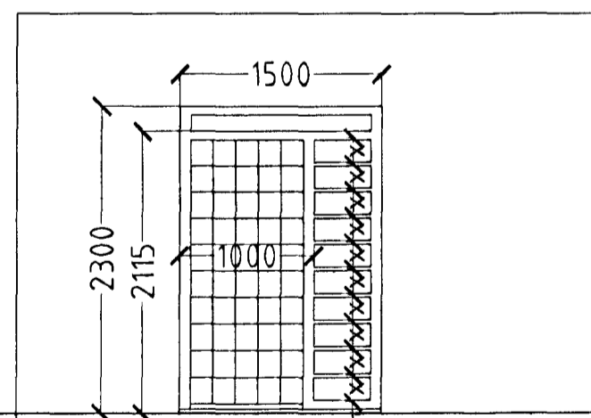
1 STK ANDD. HURÐ OP ÚT V.
