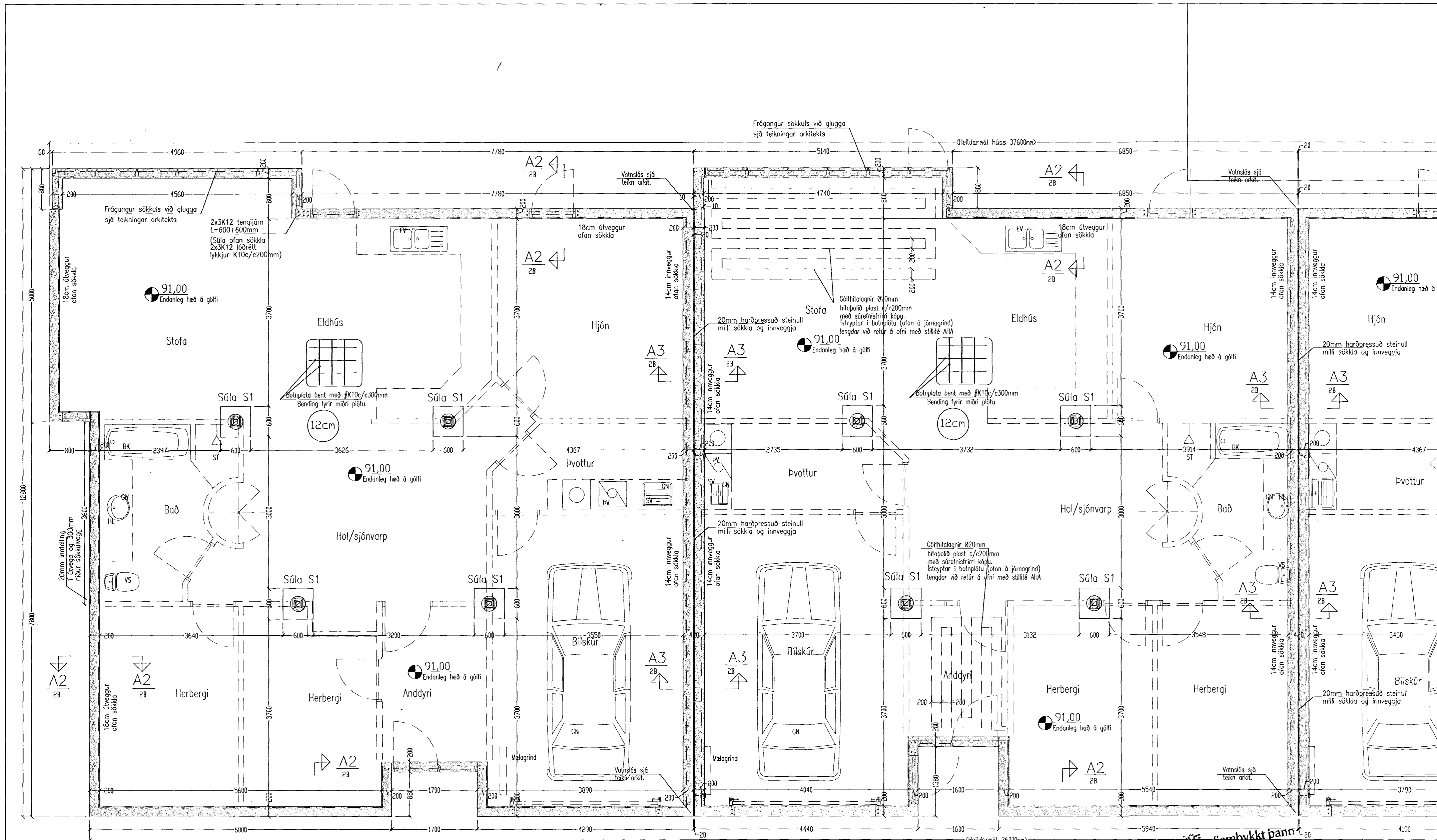
Grunnmynd sökkla 1:50 ↗ A2/2B Hús nr. 59
