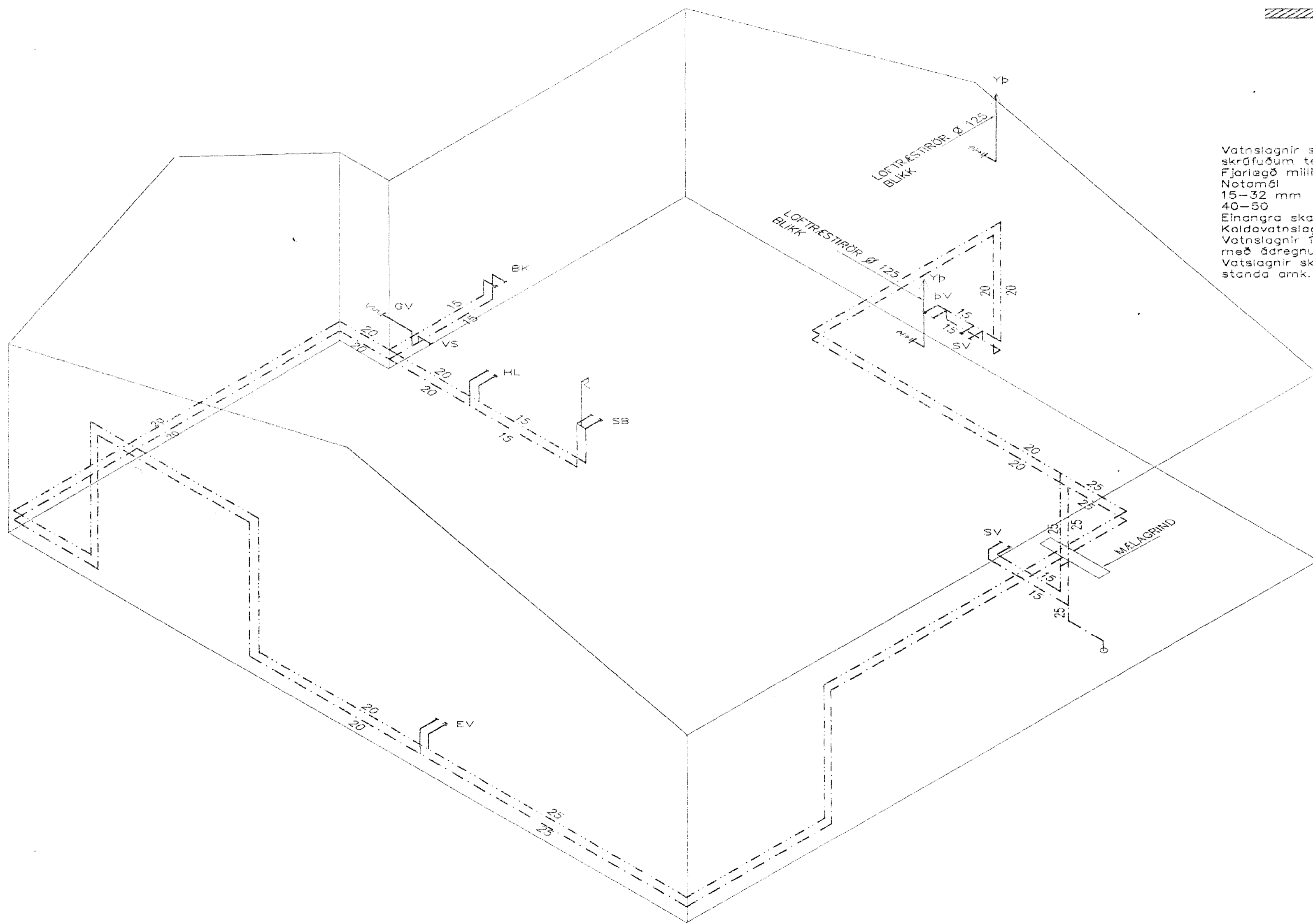
RÚMMYND VATNS OG LOFTRÆSTILAGNA 1:50
