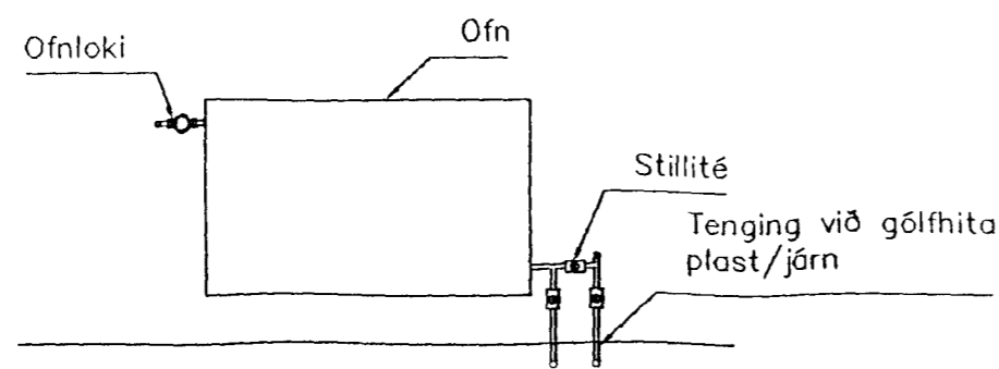
Tenging gólfhita
