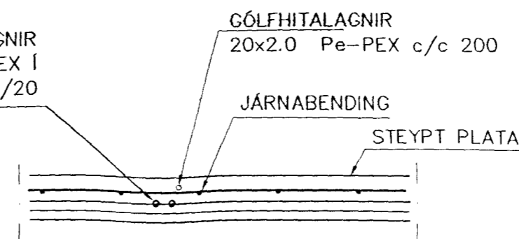
LAGNIR, SNIÐ, 1:20
