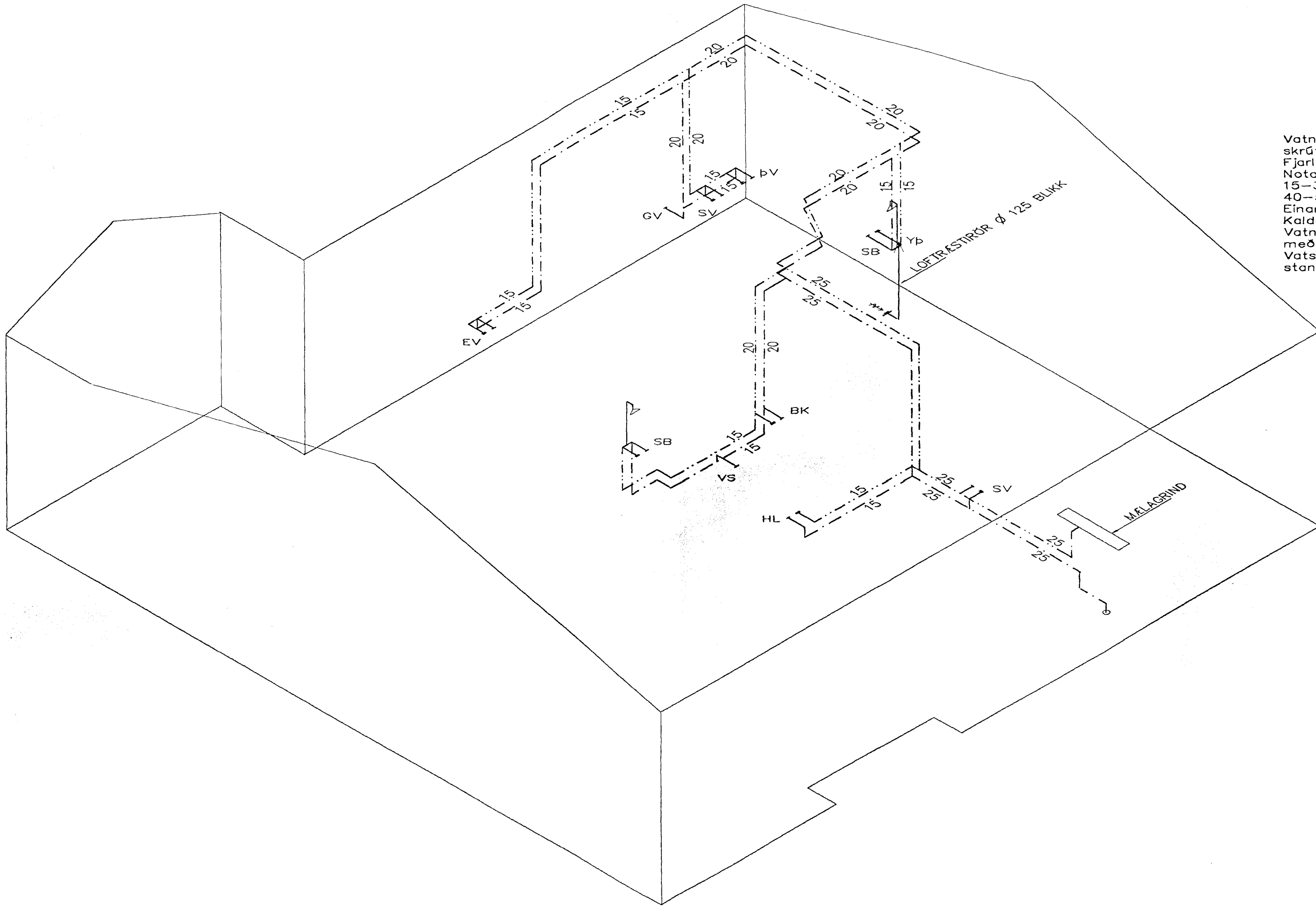
RÚMMYND VATNS OG LOFTRÆSTILAGNA 1:50
