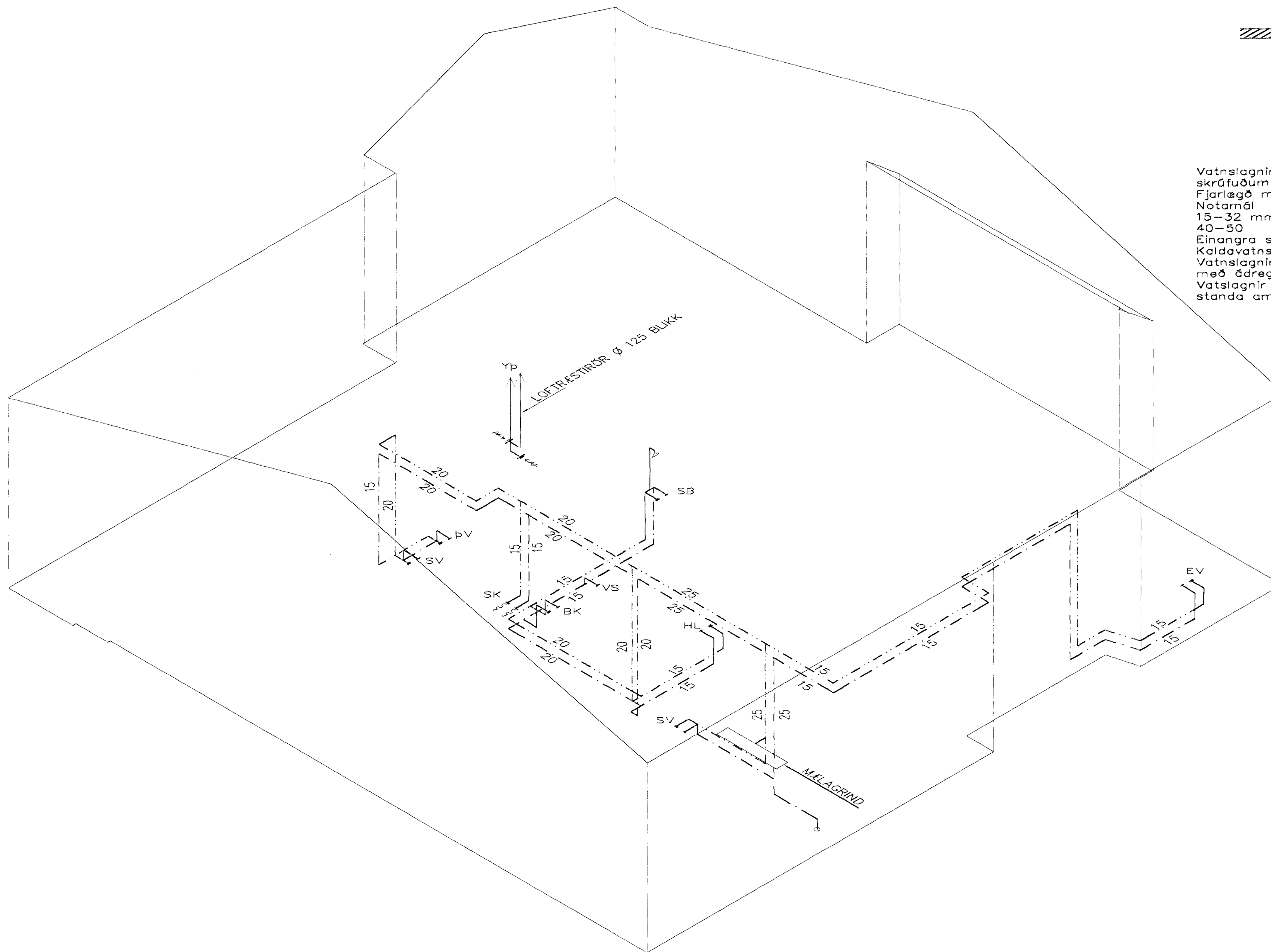
RÚMMYND VATNS OG LOFTRÆSTILAGNA 1:50
