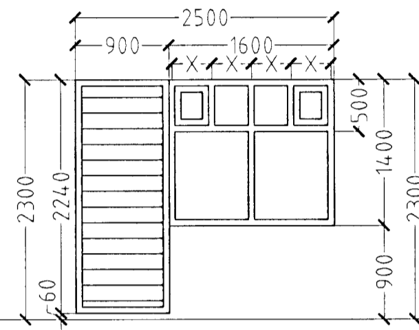
1 STK GEYMSLA
