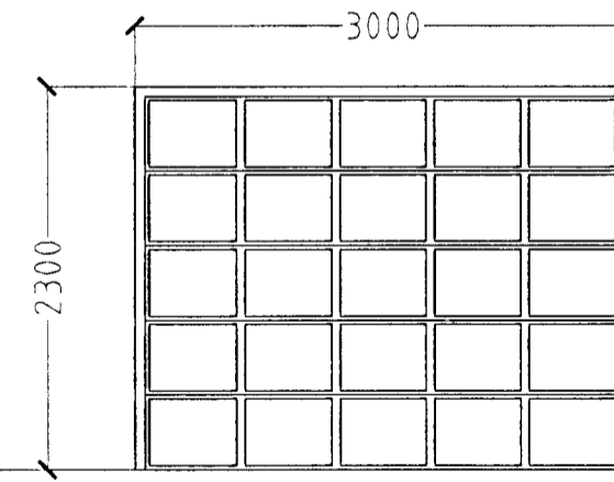
1 STK BÍLGEYMSLA
