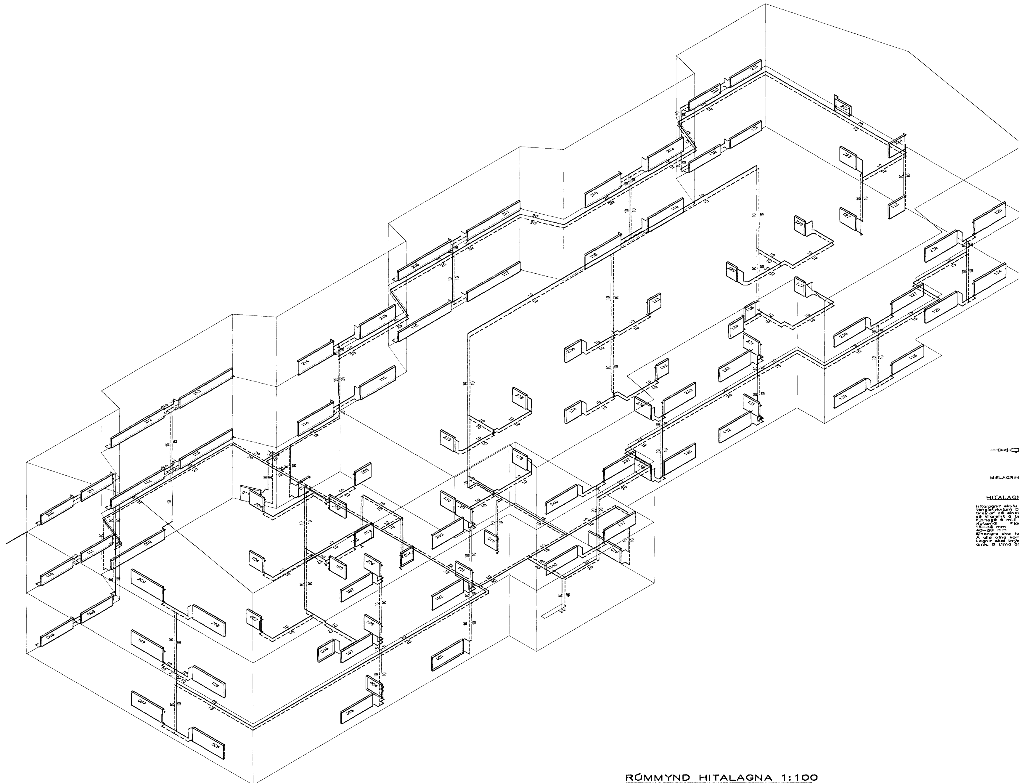
RÖMMYND HITALAGNA 1:100
