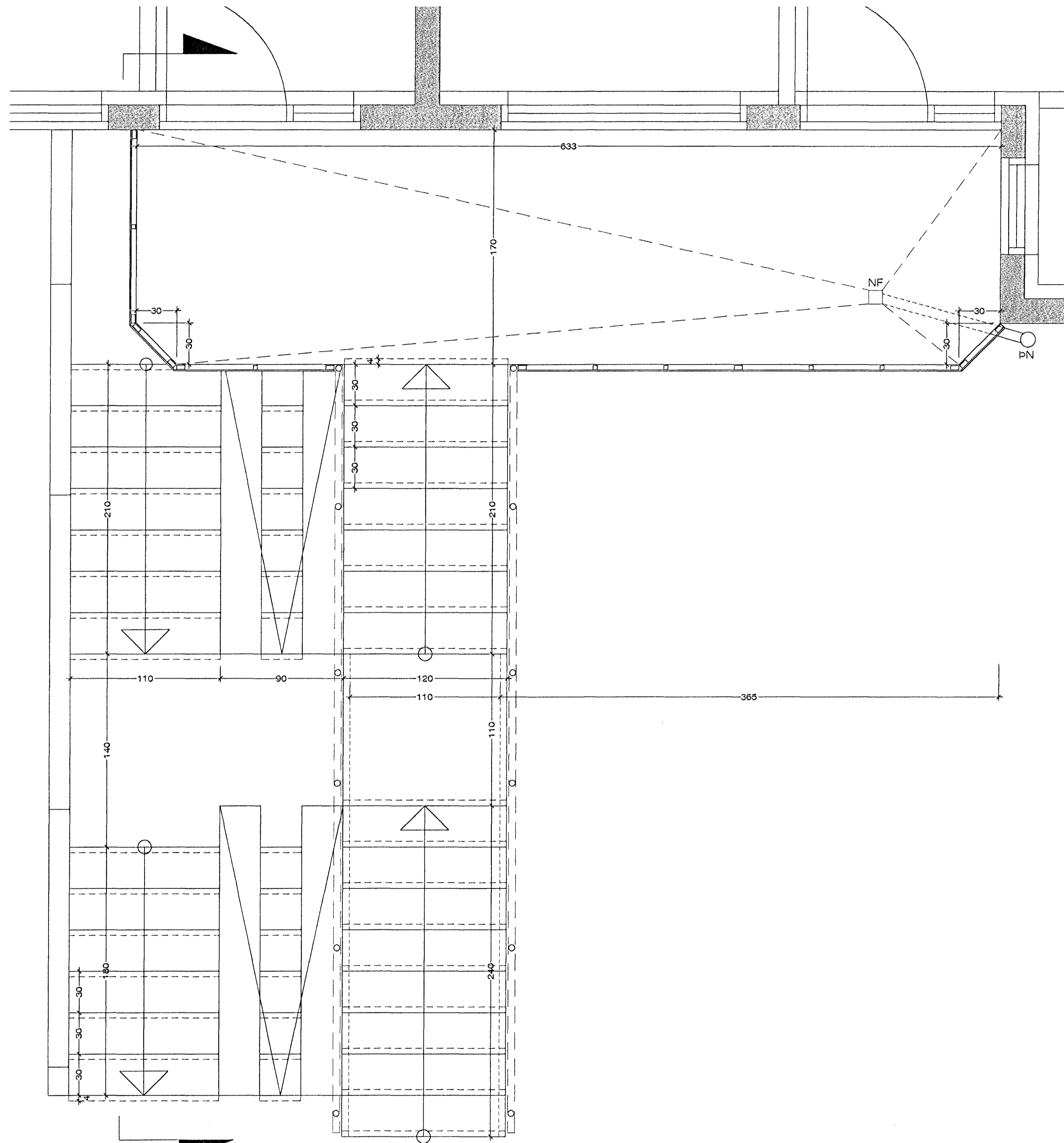
GRUNNMYND STIGA 71A M 1 : 20
