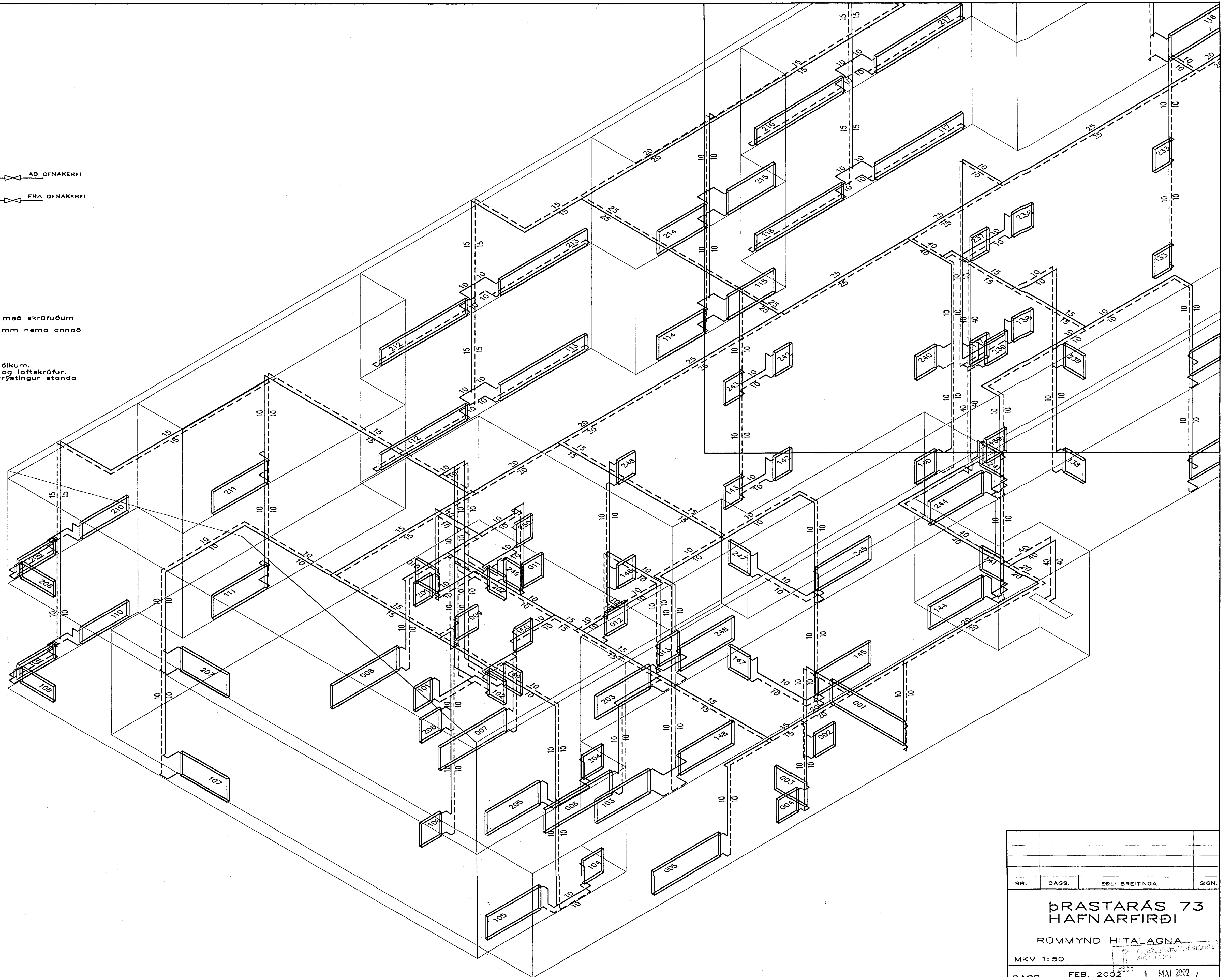
RÚMMYND HITALAGNA 1:50
