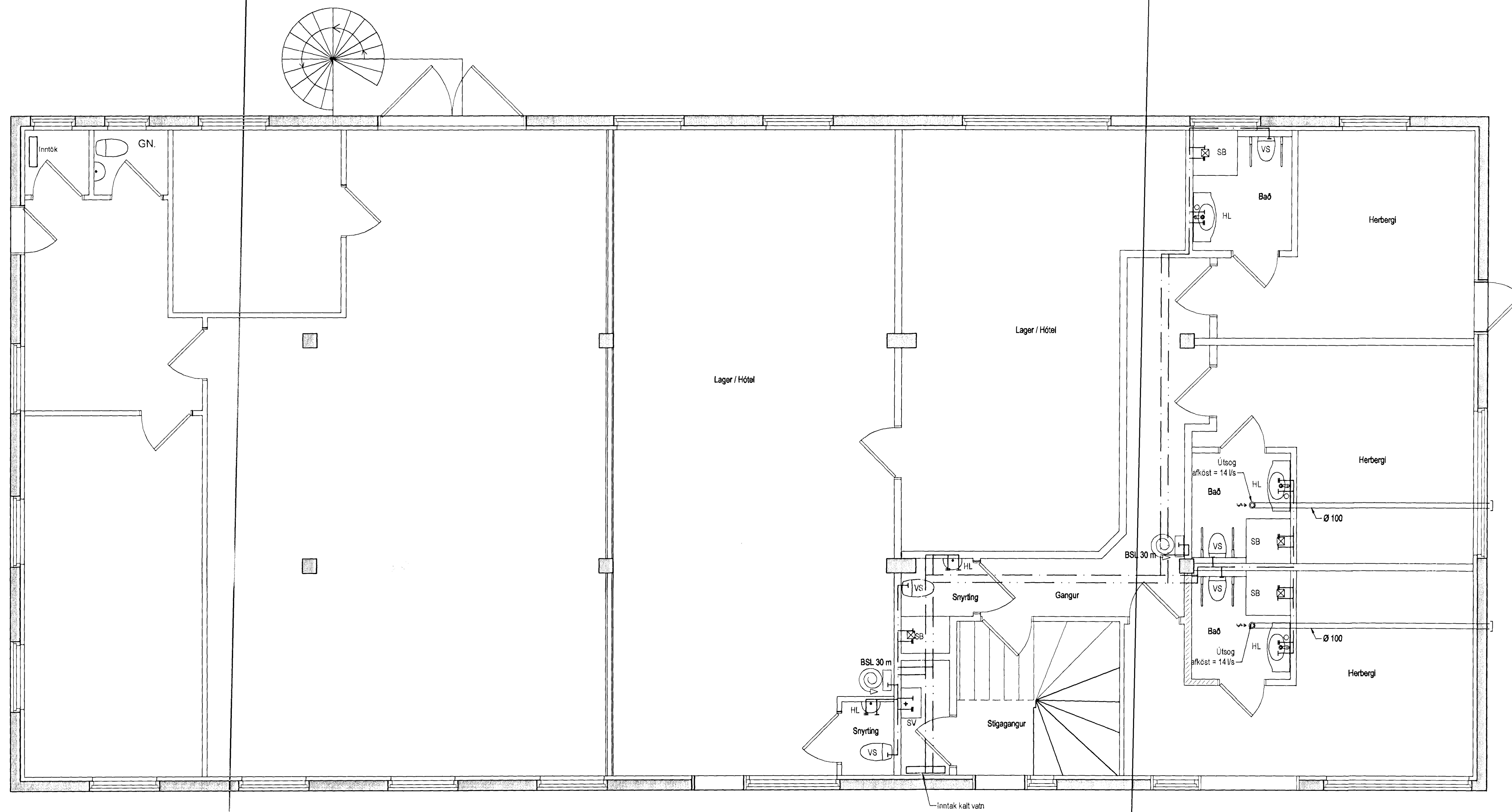
Lagnir 1. Hæð, Grunnmynd, 1:50
