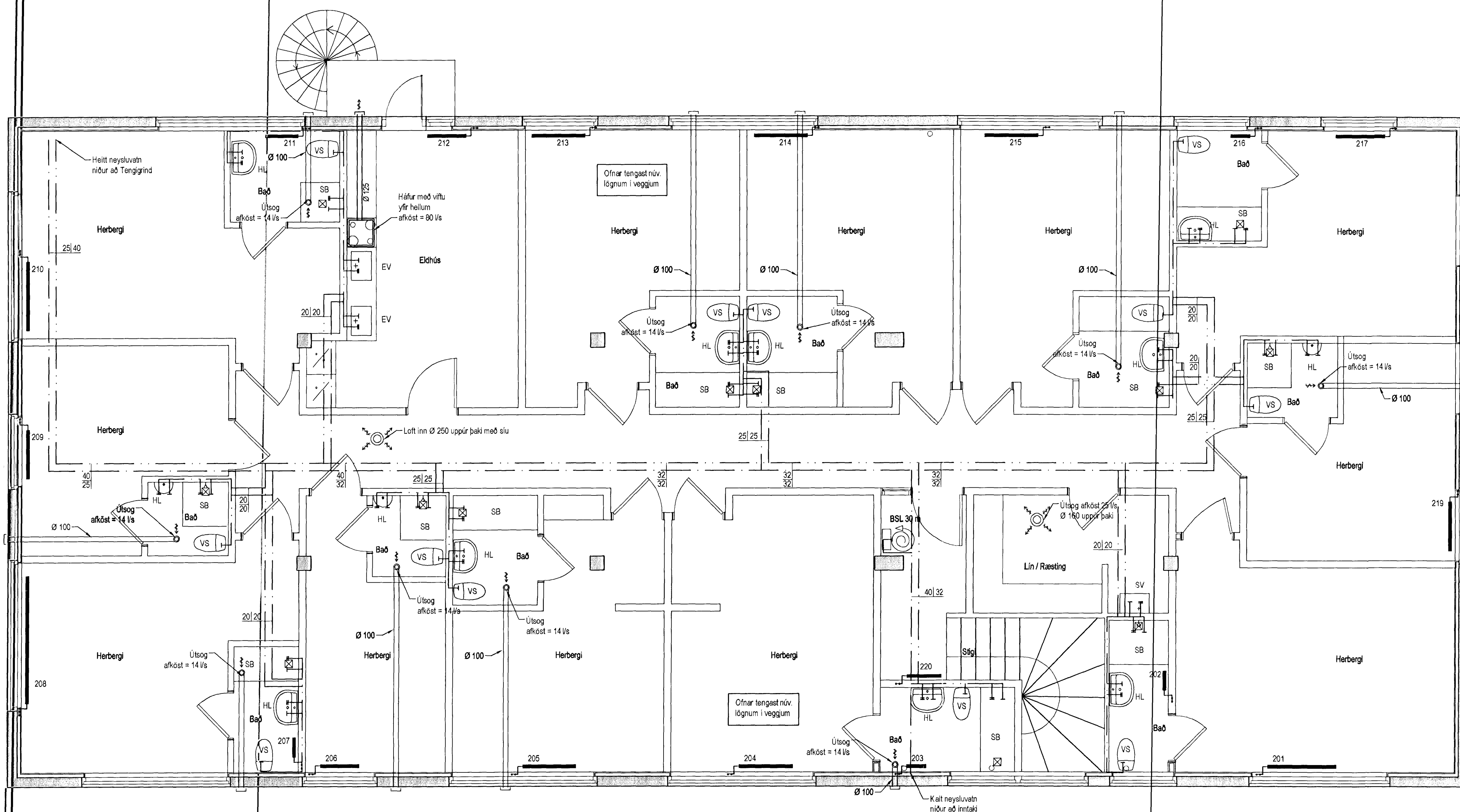
Lagnir 2. Hæð, Grunnmynd, 1:50
