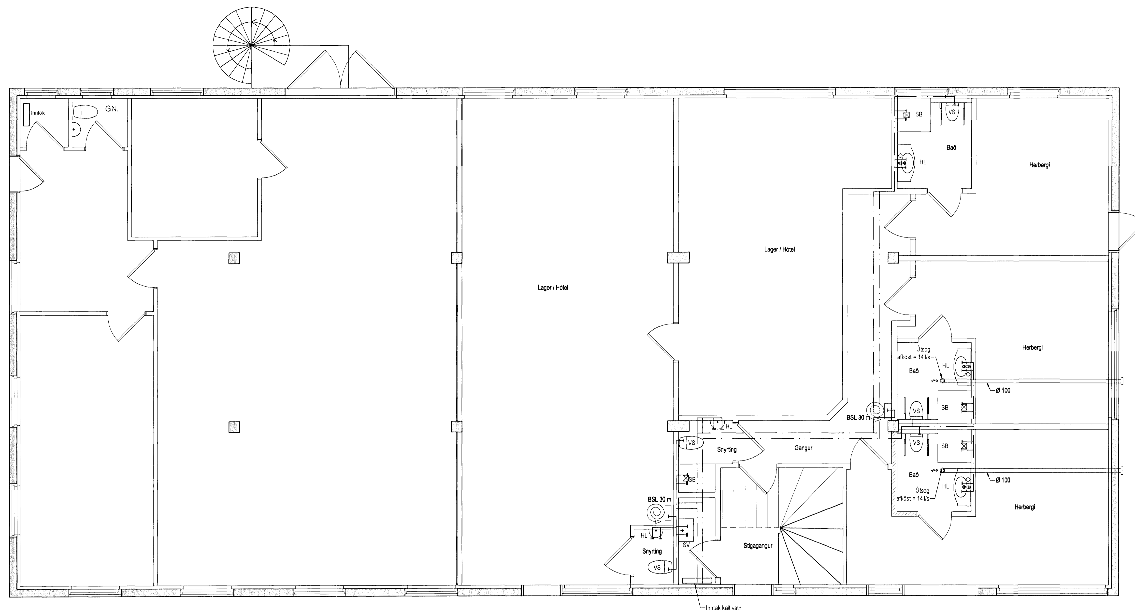
Lagnir 1. hæð, Grunnmynd, 1:50
