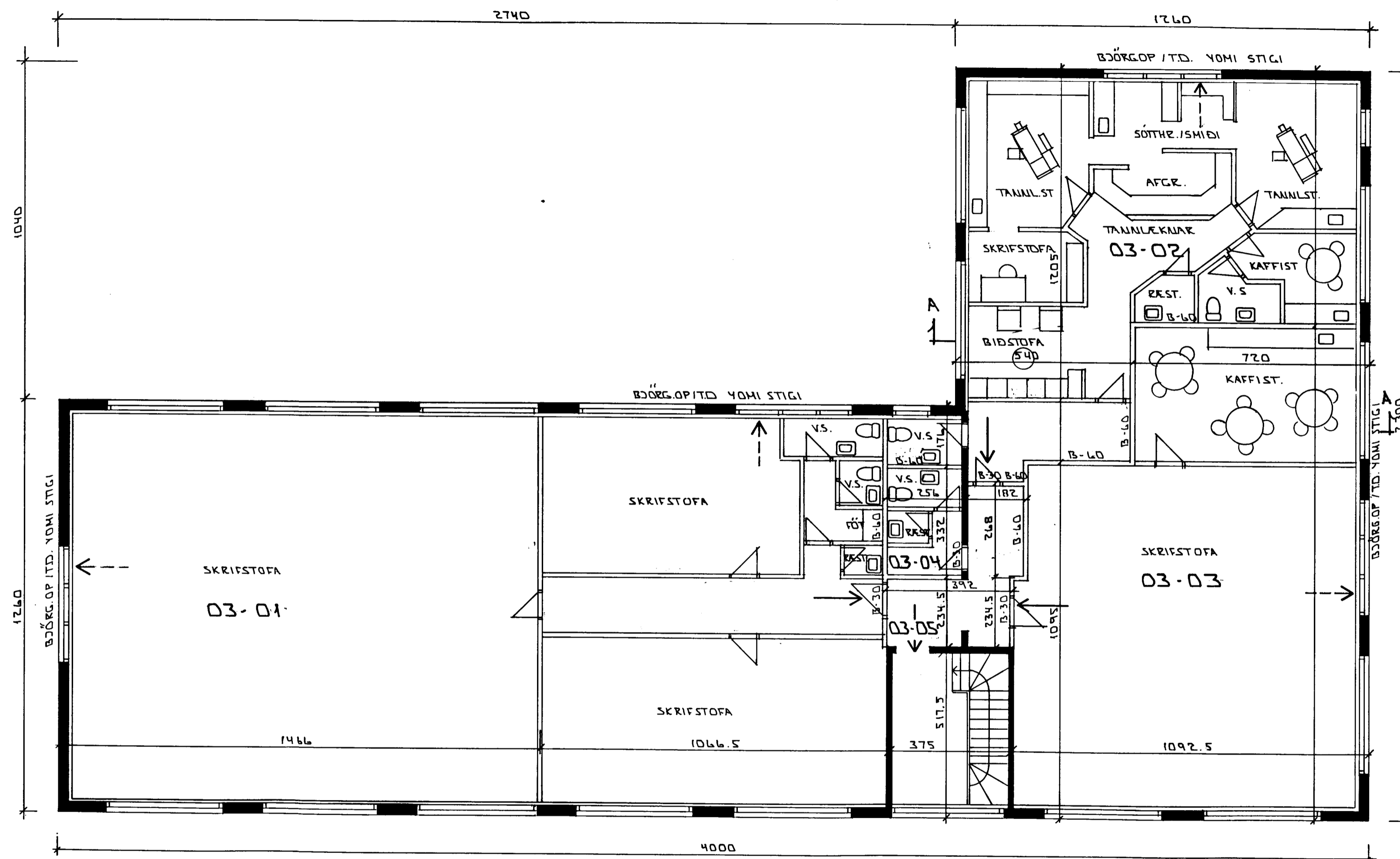
GRUNNMÝND 3. HÆÐ 1:100
