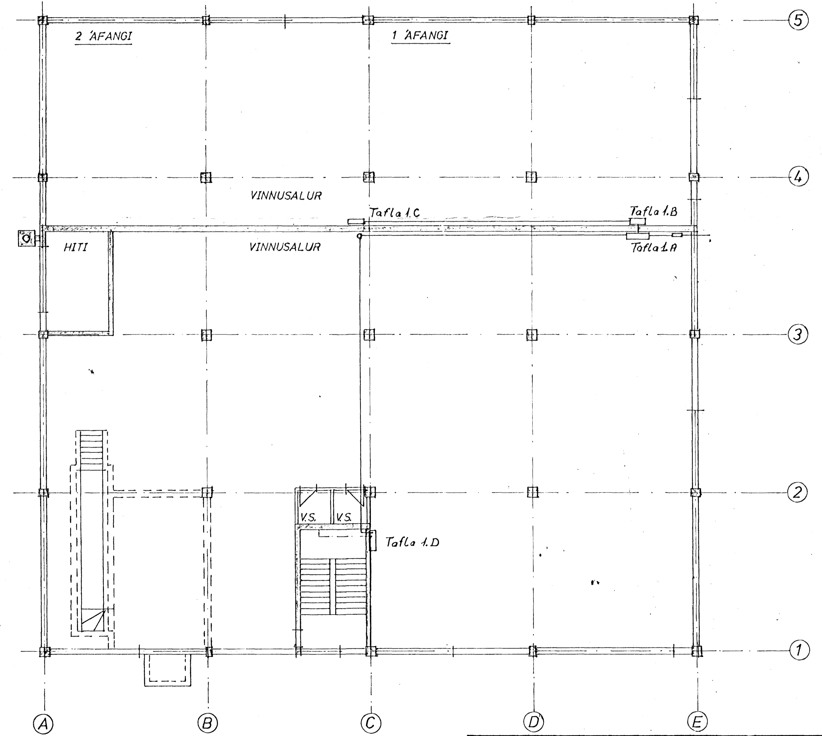
GRUNNMÝND 1 HÆÐ M 1:100
