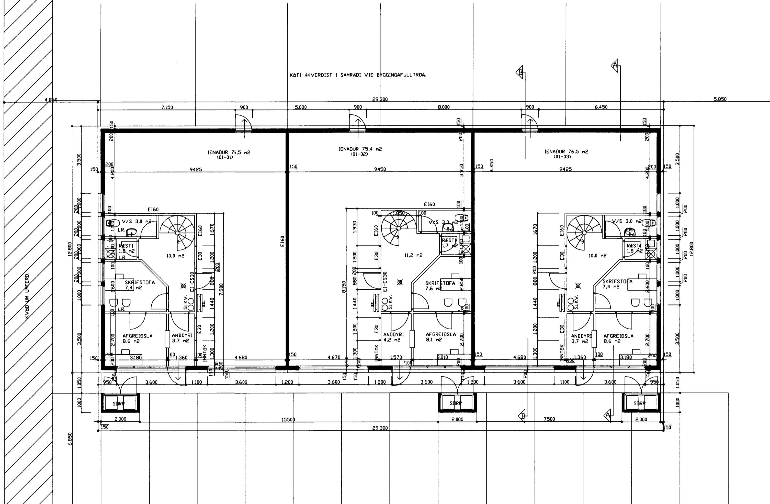
GRUNNMYND 1 HÆÐ MKV. 1:100.
