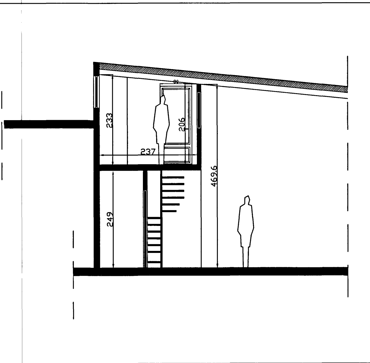
SKURDMYND A-A MVK 1/20
