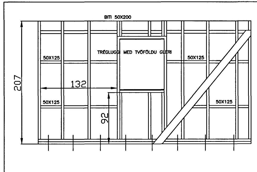
VIDAR VEGGUR ( KAFFISTOFA ) MVK 1/20
