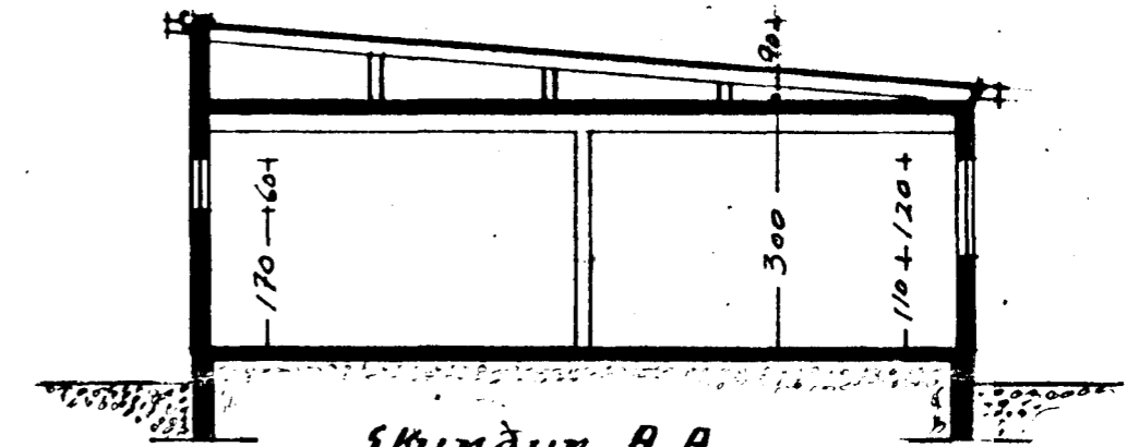
Skurður AA
