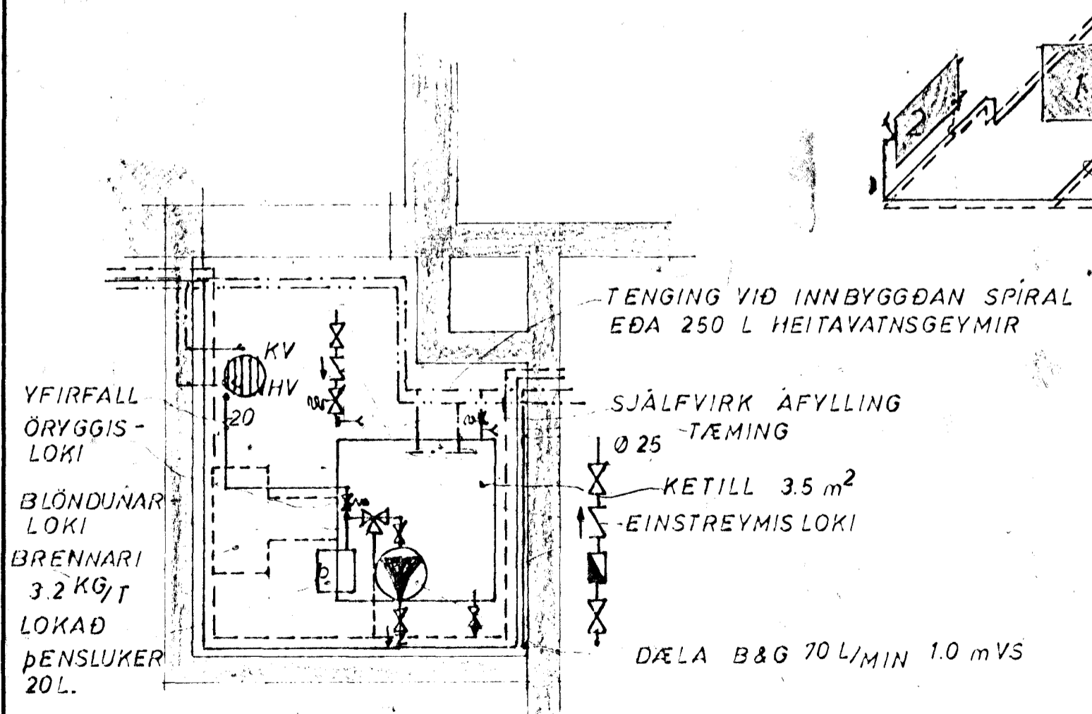
GRUNNMYND HITAKLEFA ~ 1:20
