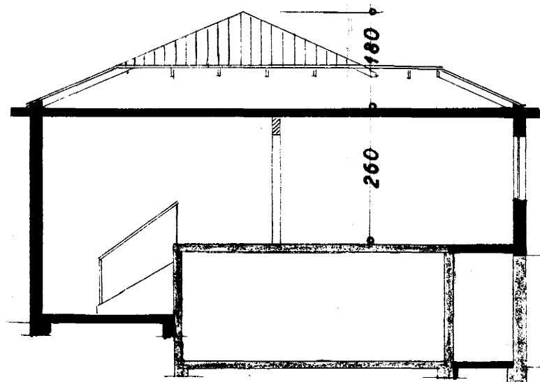
Snið: A
