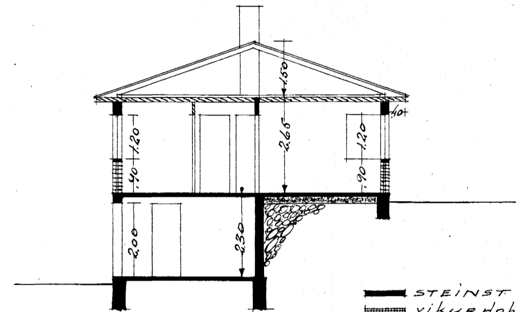
SKURÐUR A-B
