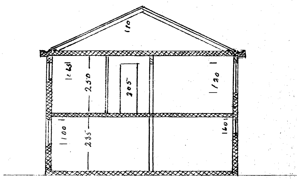
Þverskurður A-B
