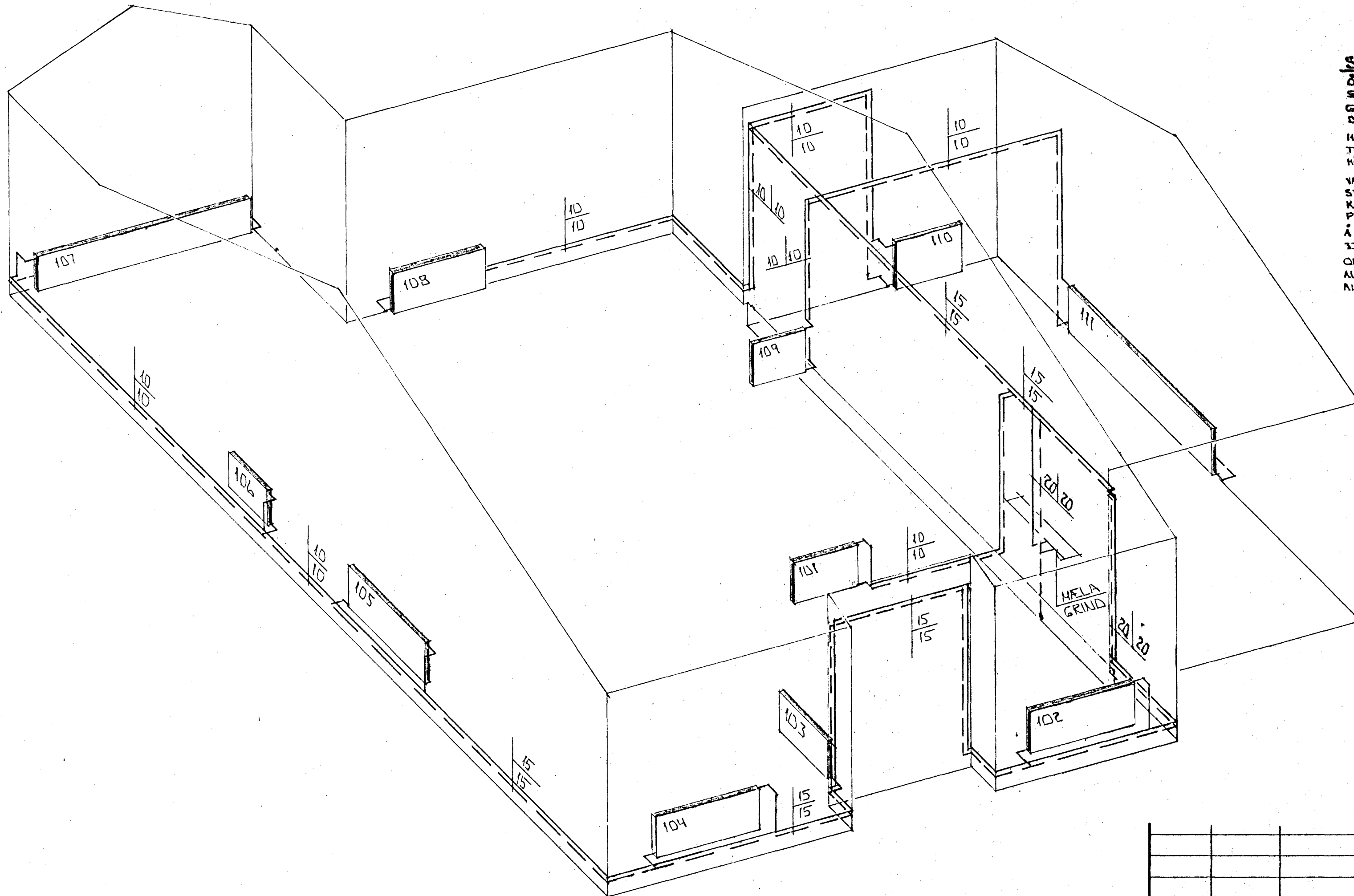
RÚMMYND 1:50
