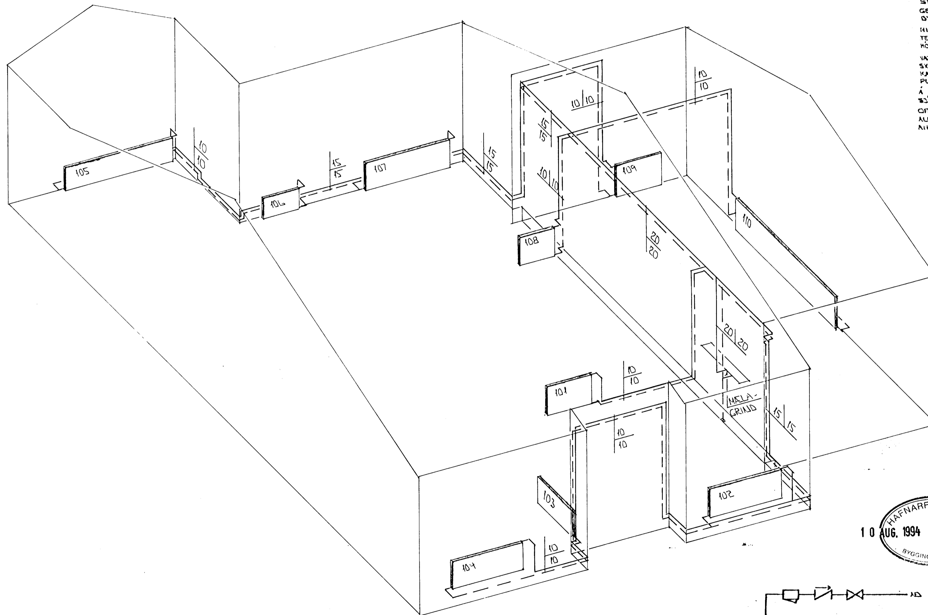
RÚMMYND - HITALAGNA 1:50
