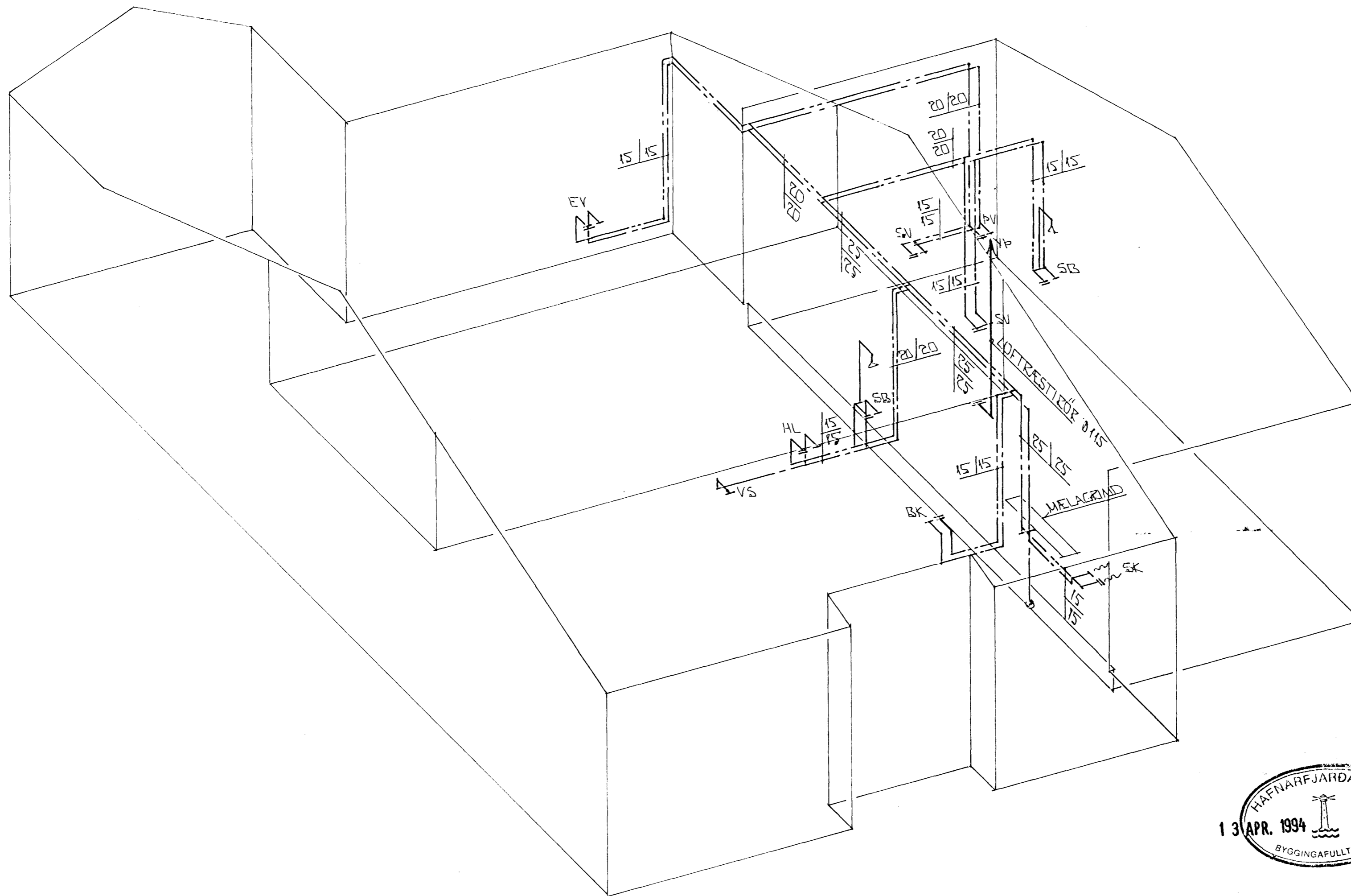
RÚMMYND VATNSLAGNA 1:50
