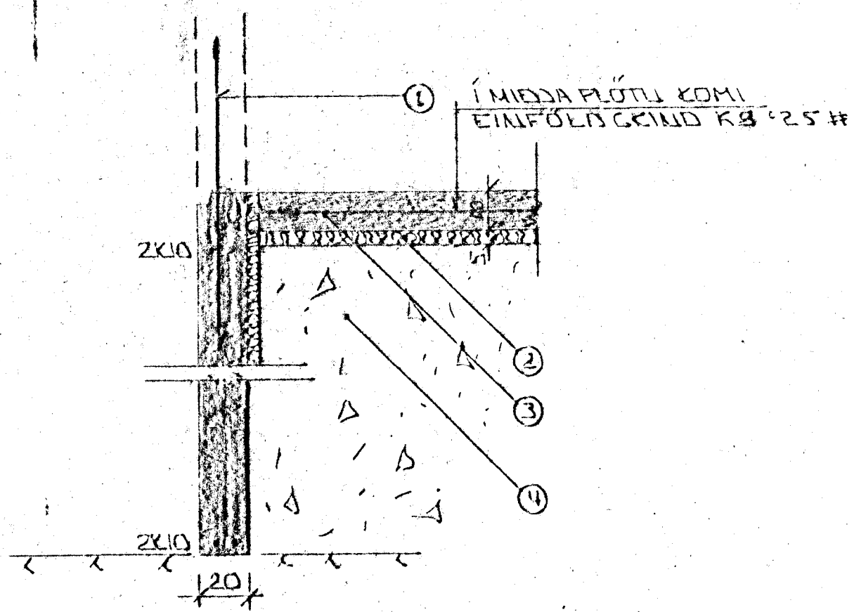
SNID 1 Í ÚTVEGGI 1:20
