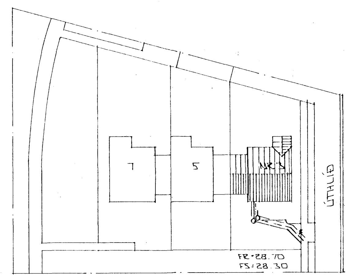
AFSTÖÐUMYND 1:500
