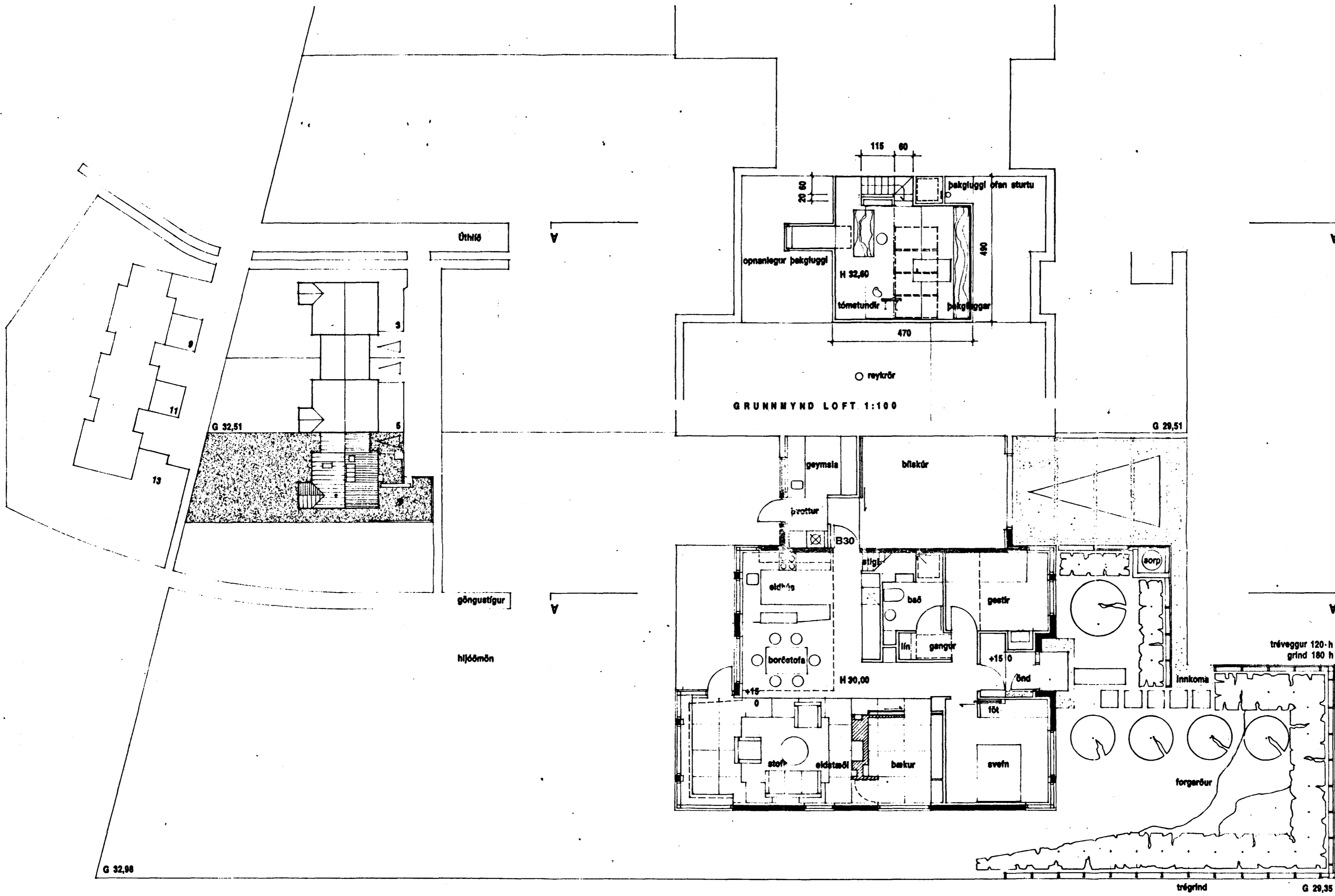
AFSTÖÐUMYND 1:500
