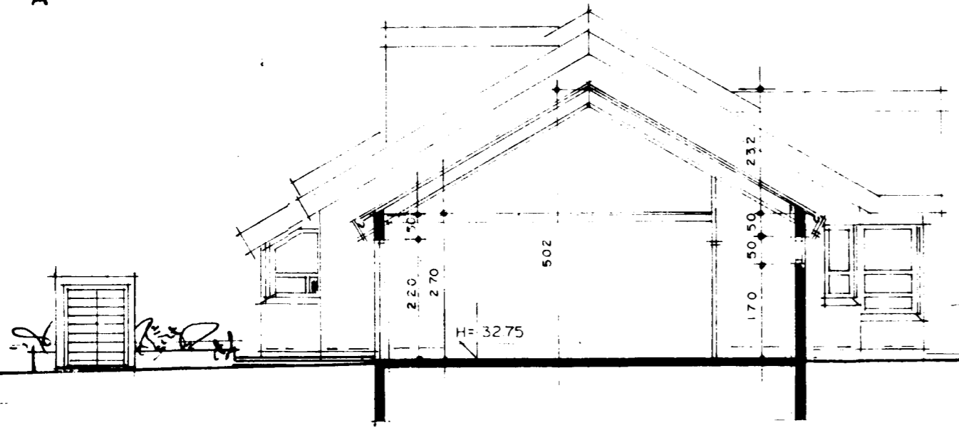
SNEIÐING B-B
