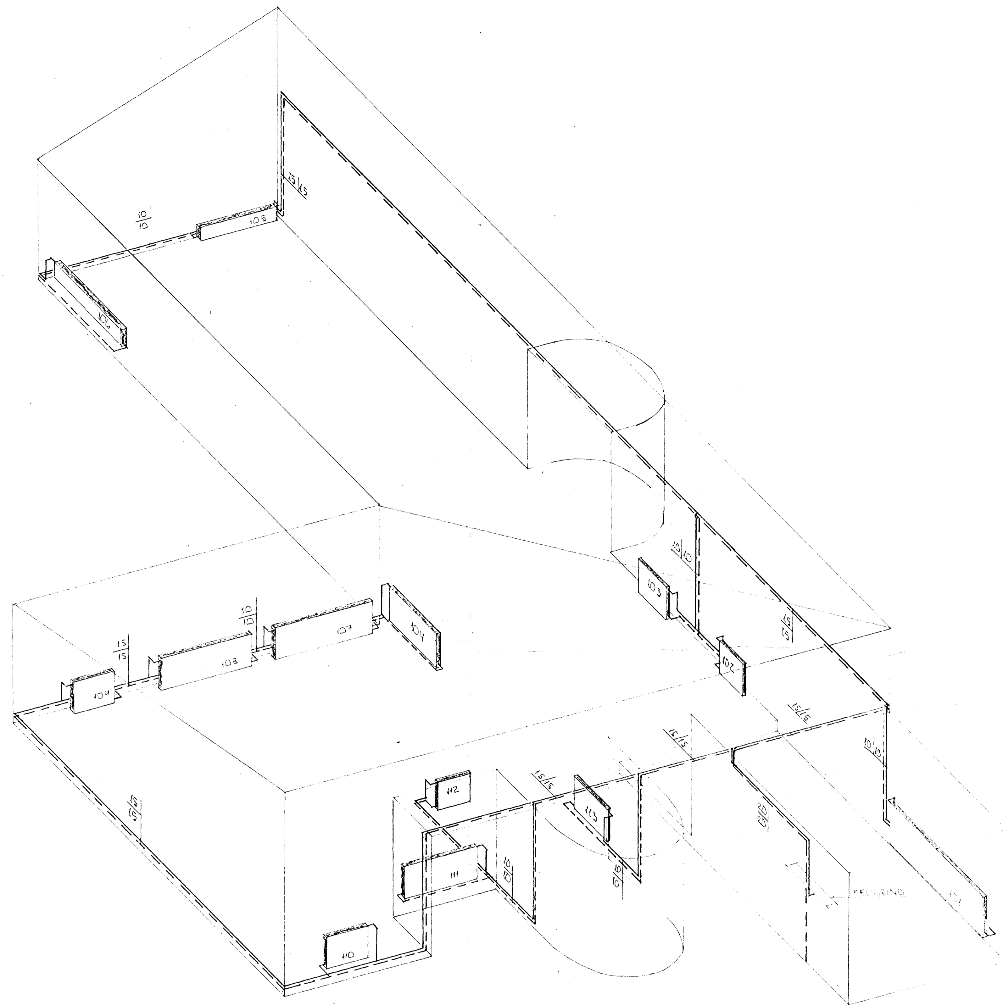
RÚMMYND HITALAGNA 1:50
