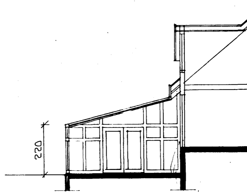
SNJID A-A • 1:100
