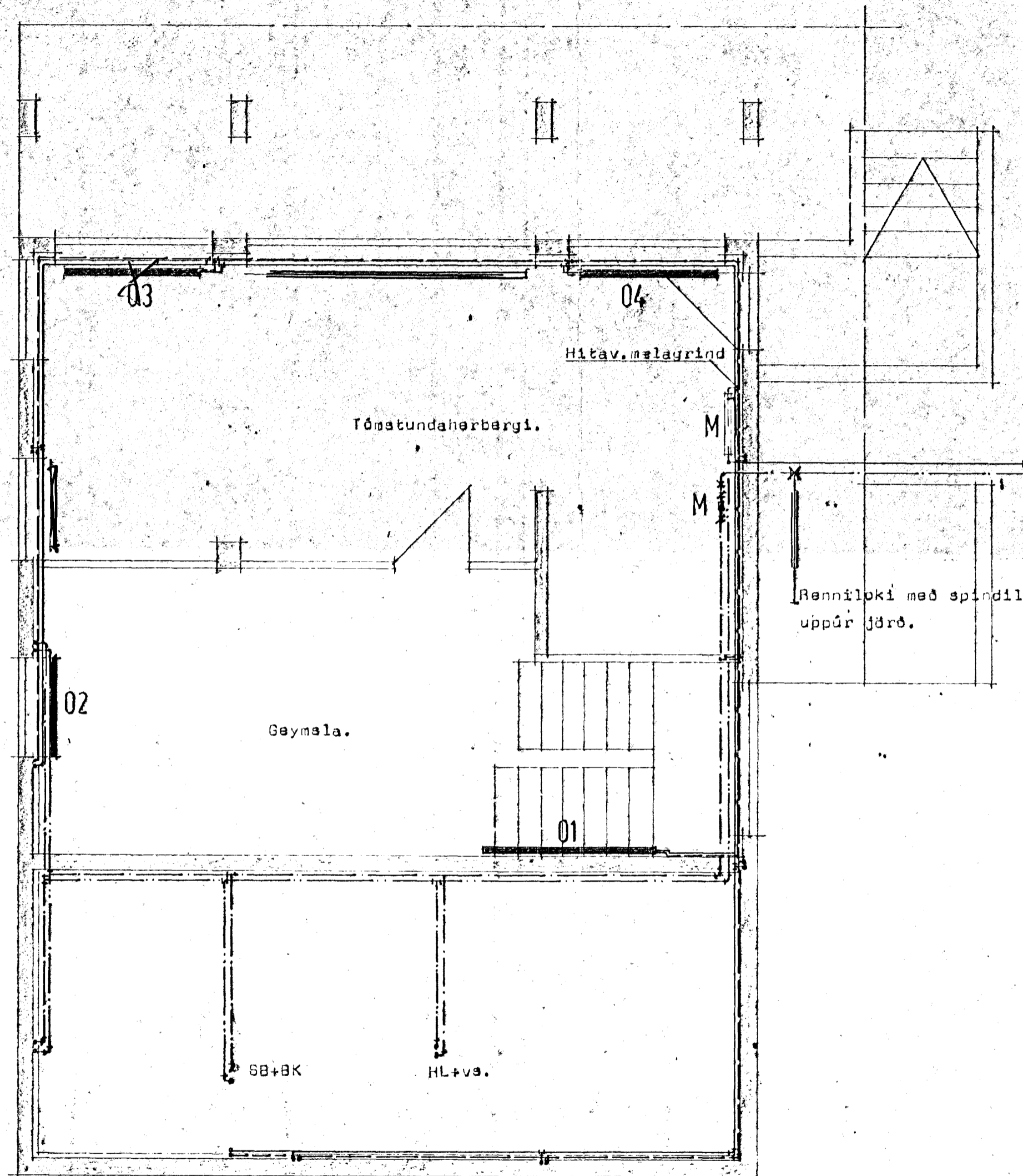
Grunnmynd Kjallara mk 1:50
