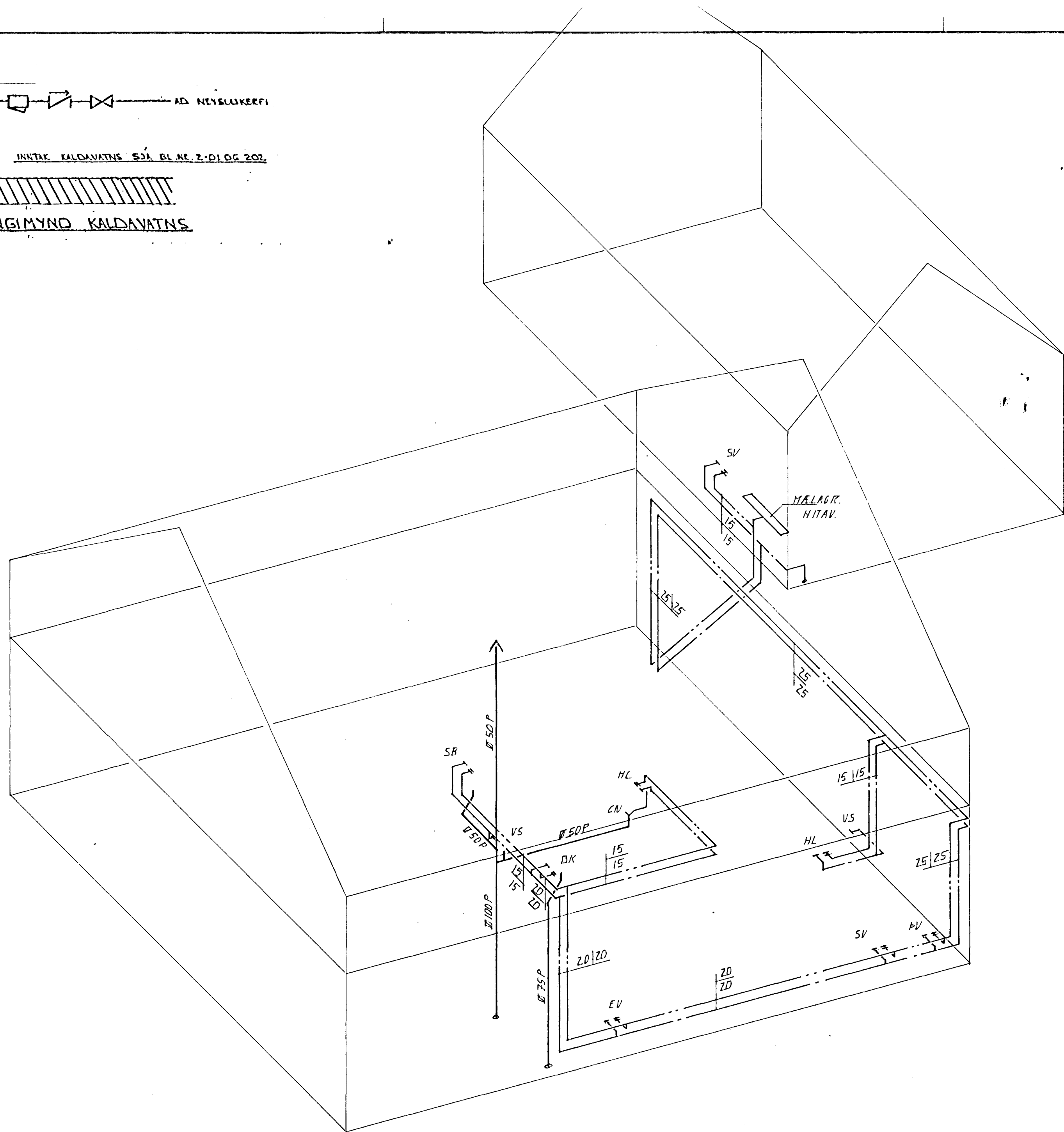
VATNS- OG FRÁRENNSLISLAGNIR RÚMMYND, 1:50
