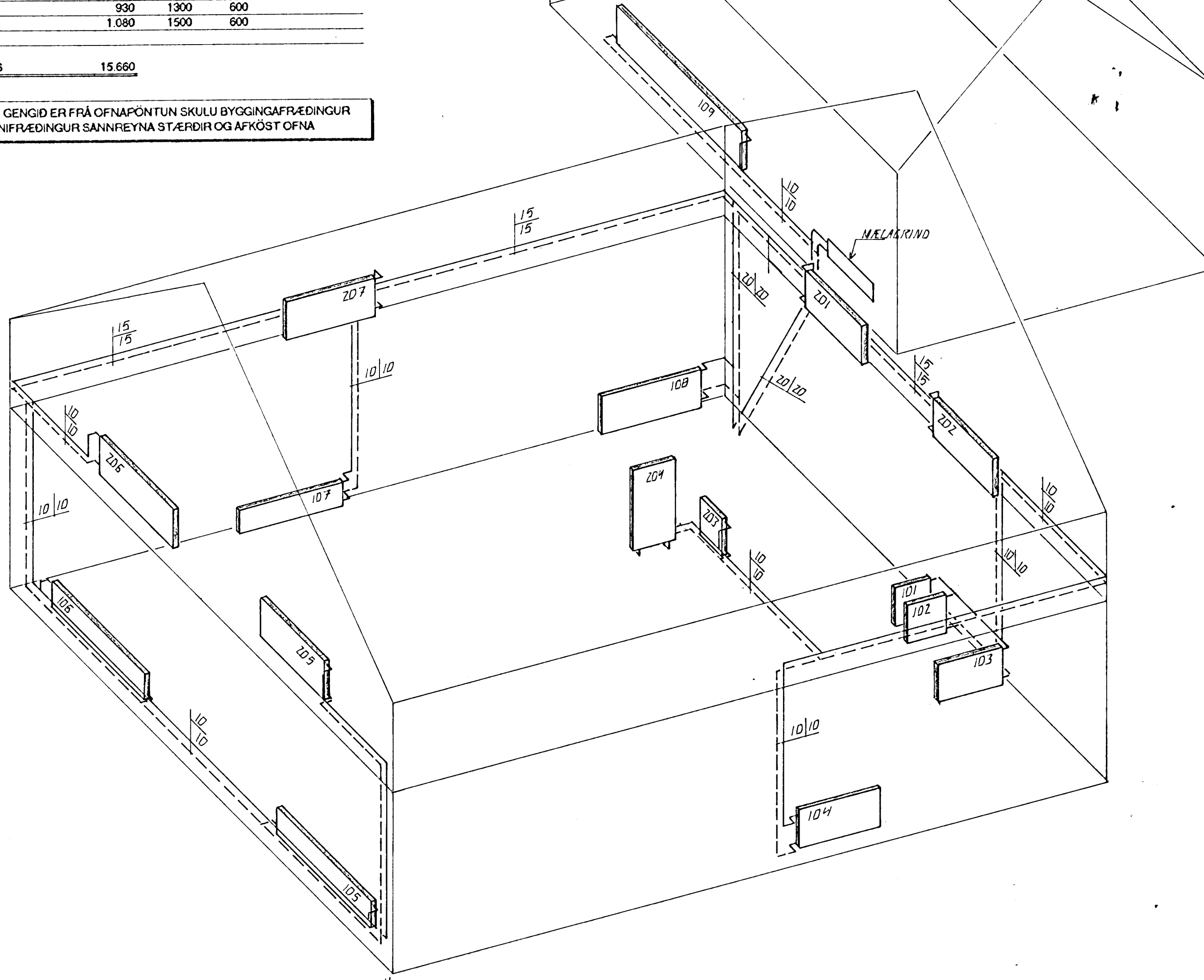
HITALAGNIR . RÚMMYND . 1:50
