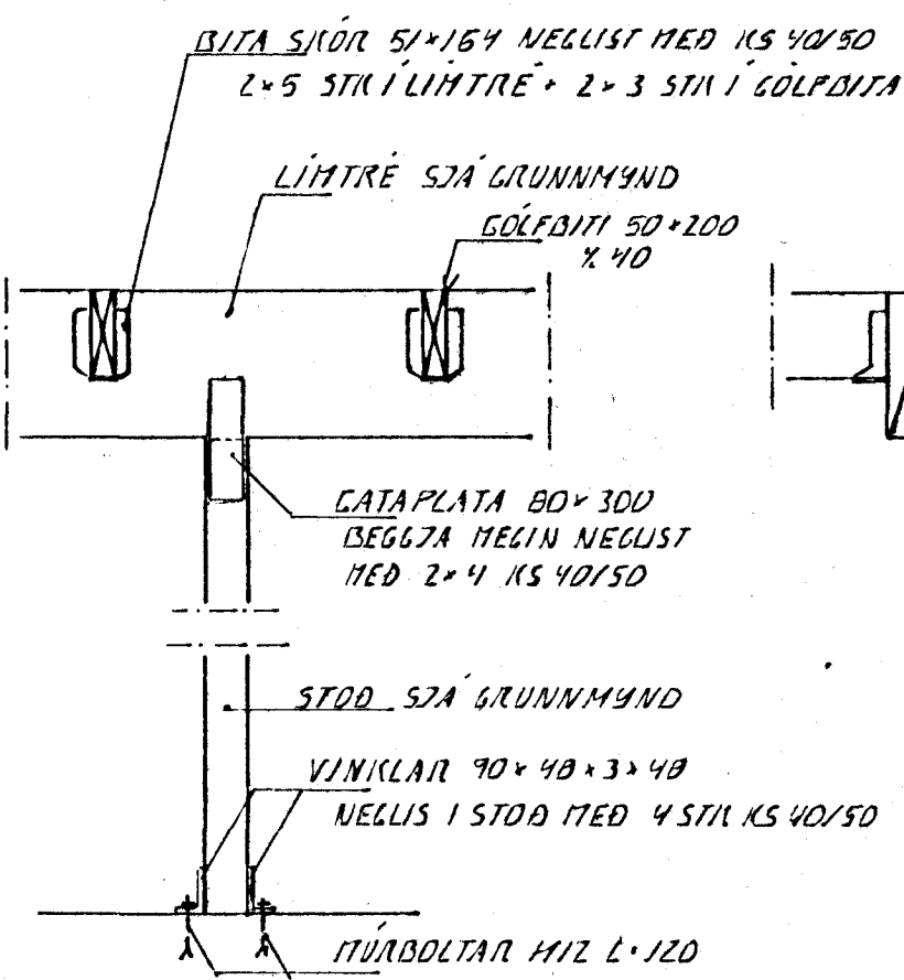
SNID 2. 1:20
