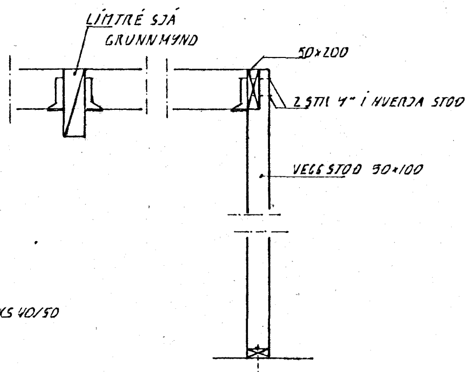
SNID 3. 1:20
