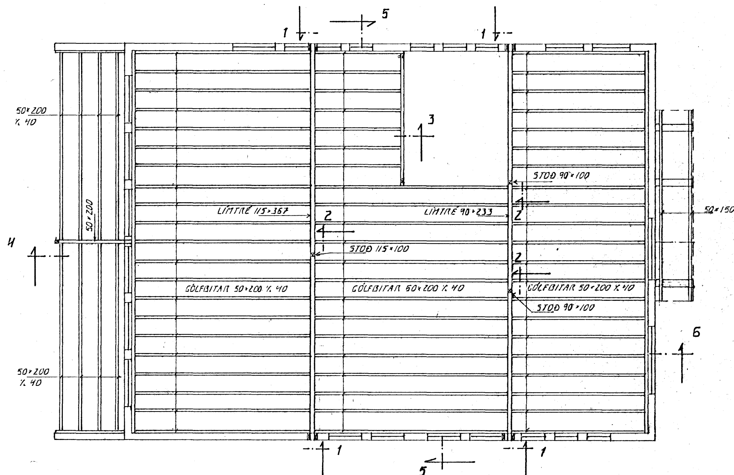
GRUNNMYND MILLI GÓLF. 1:50
