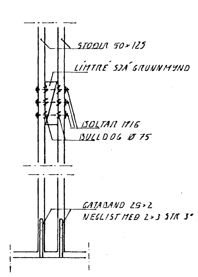
SNID 1. 1:20
