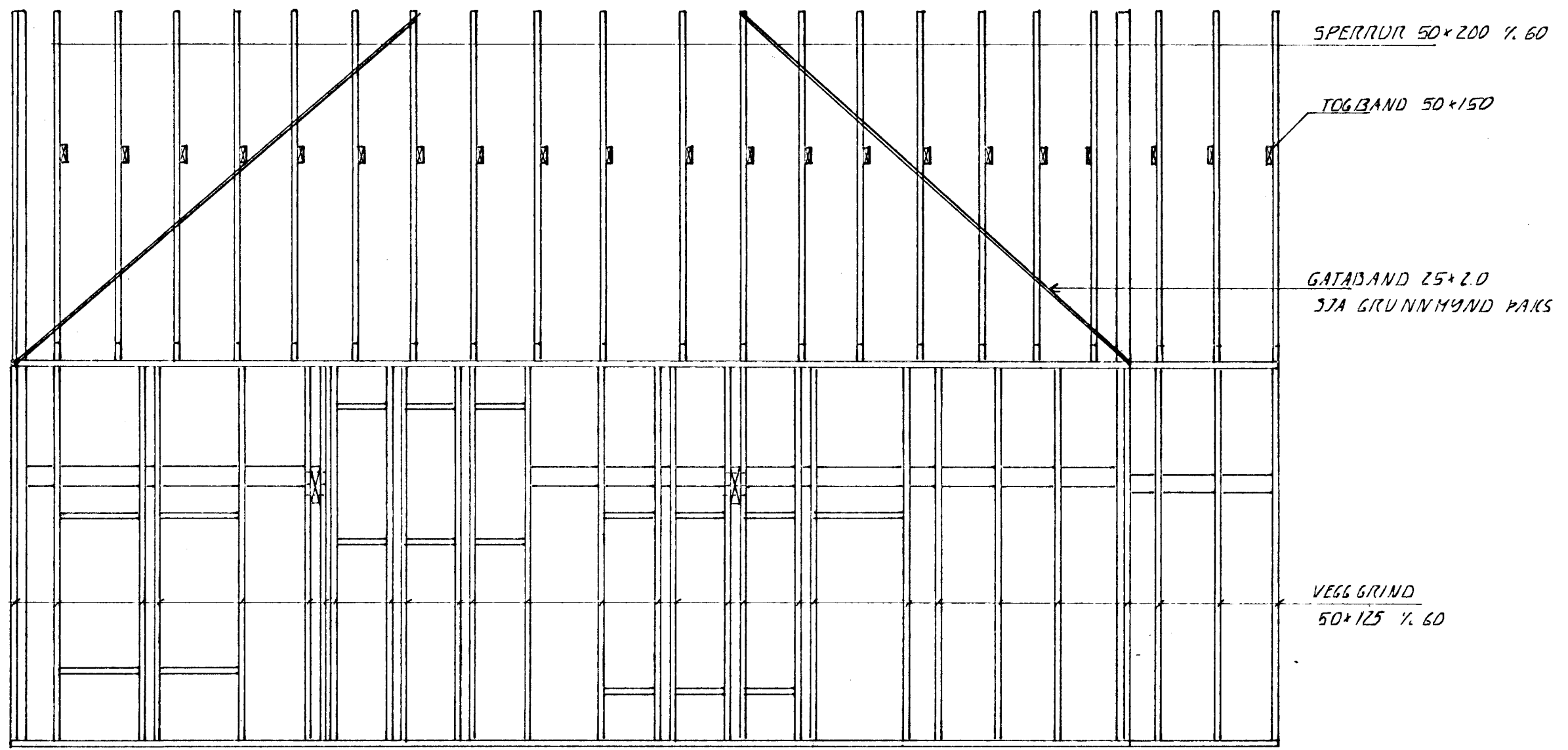
ÁSYND S-VESTUR · 1:50
