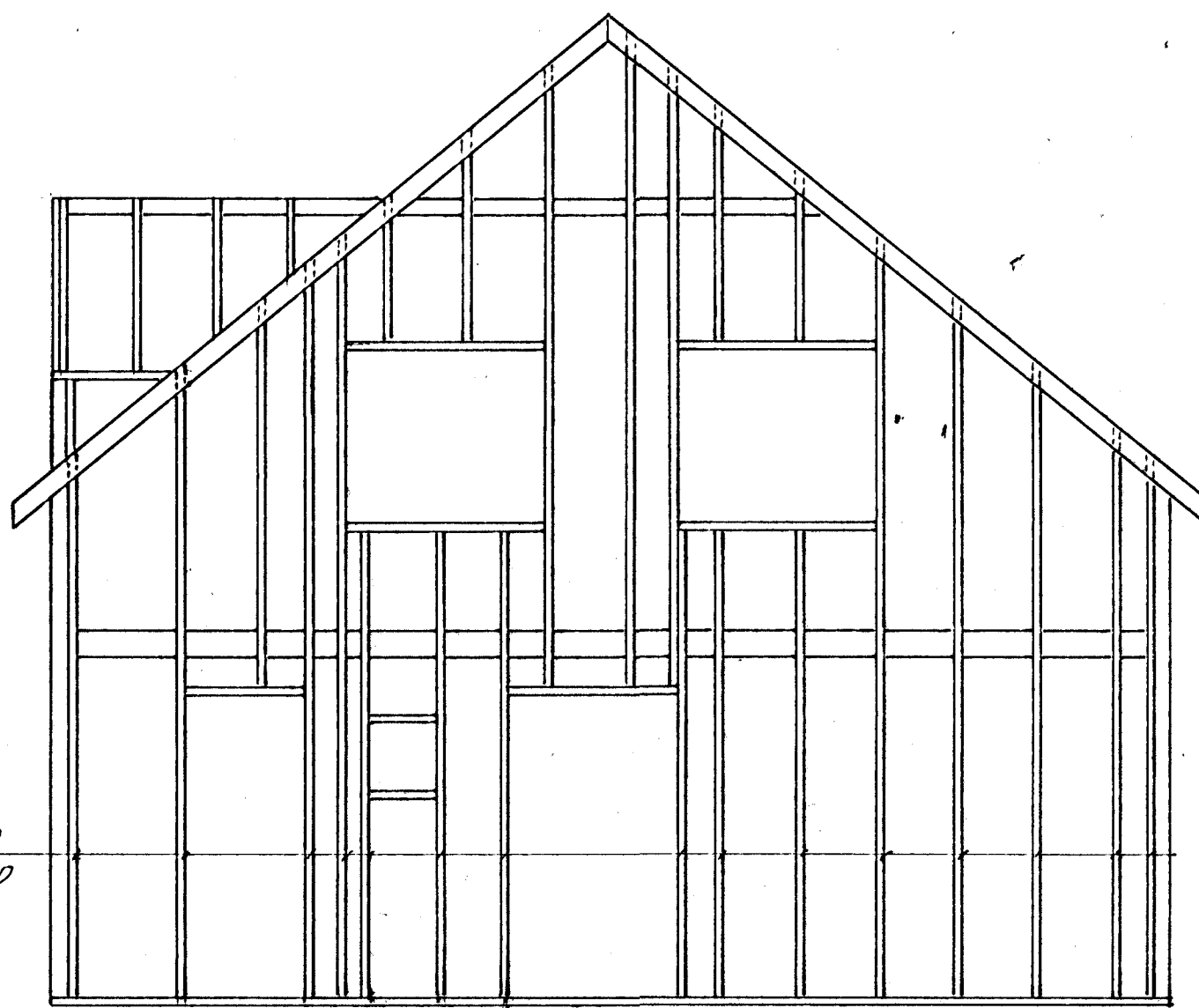
ÁSYND N-VESTUR · 1:50
