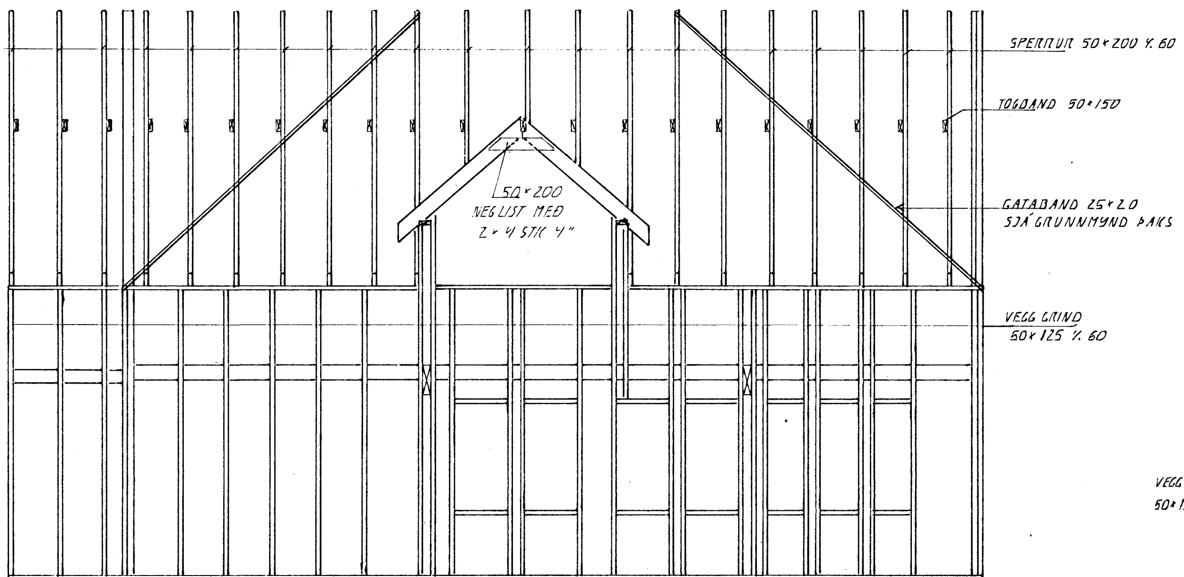
ÁSYND N-AUSTUR · 1:50
