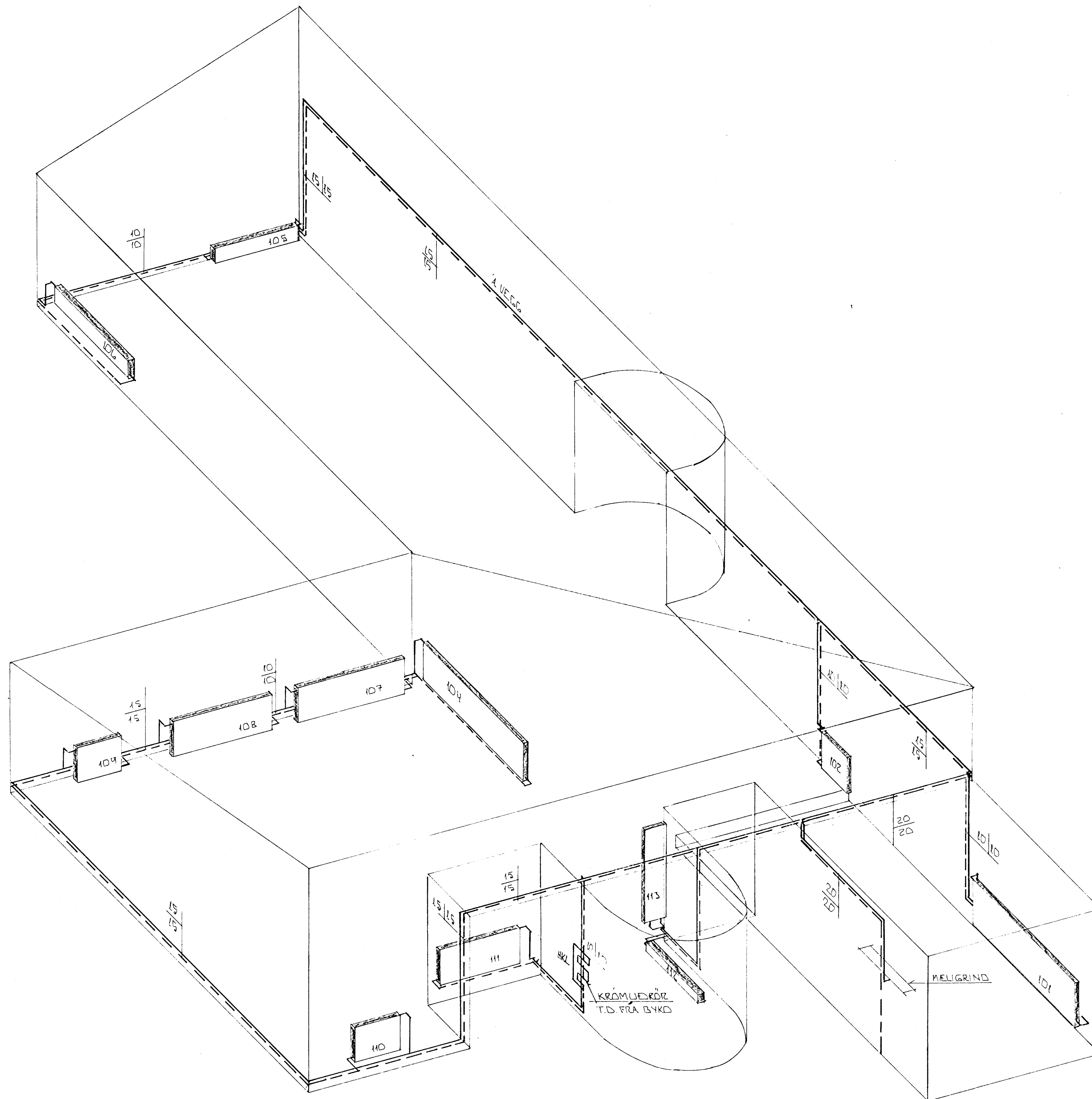
RÖMMYND HITALAGNA. 1:50
