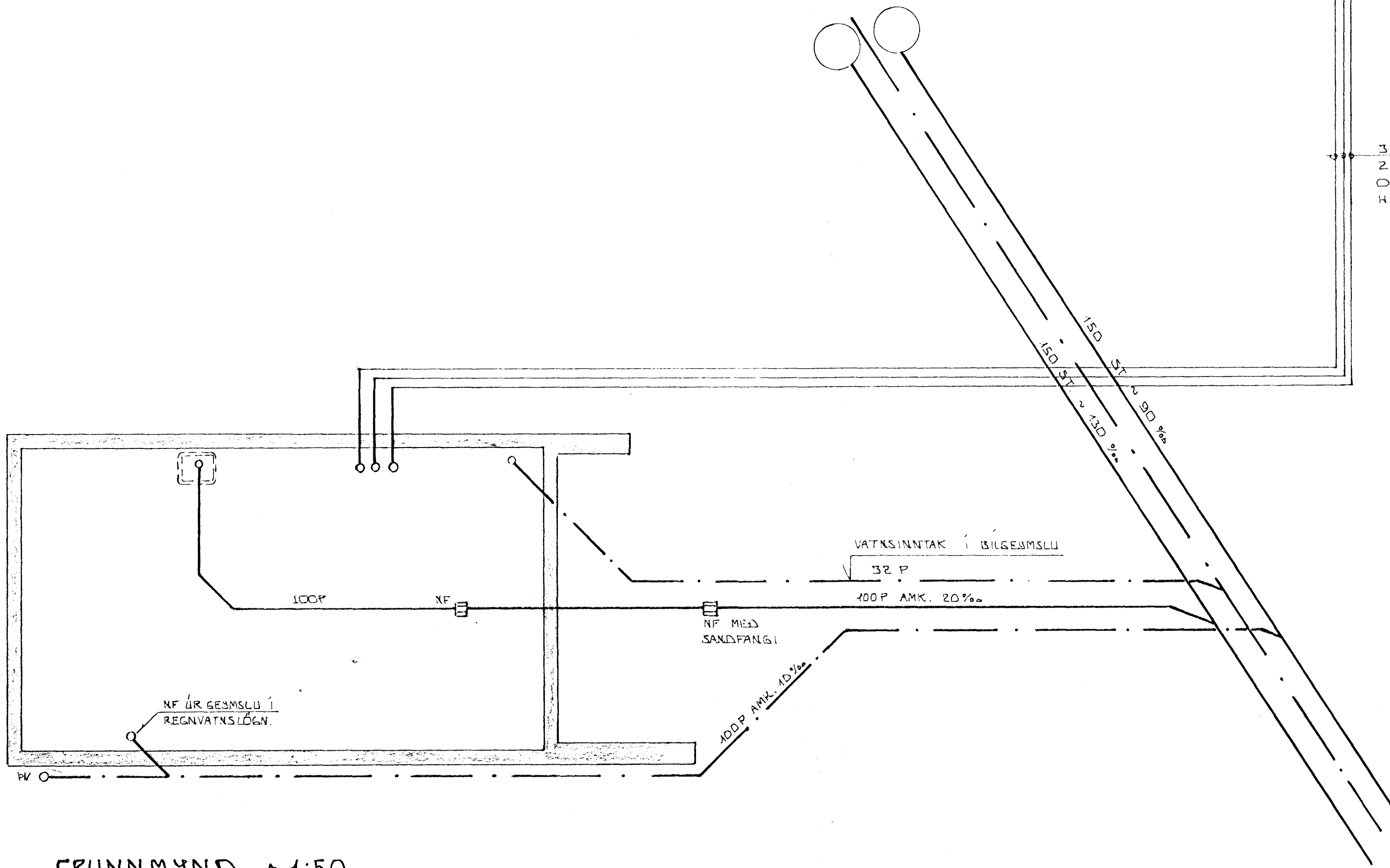
GRUNNMYND ~ 1:50
