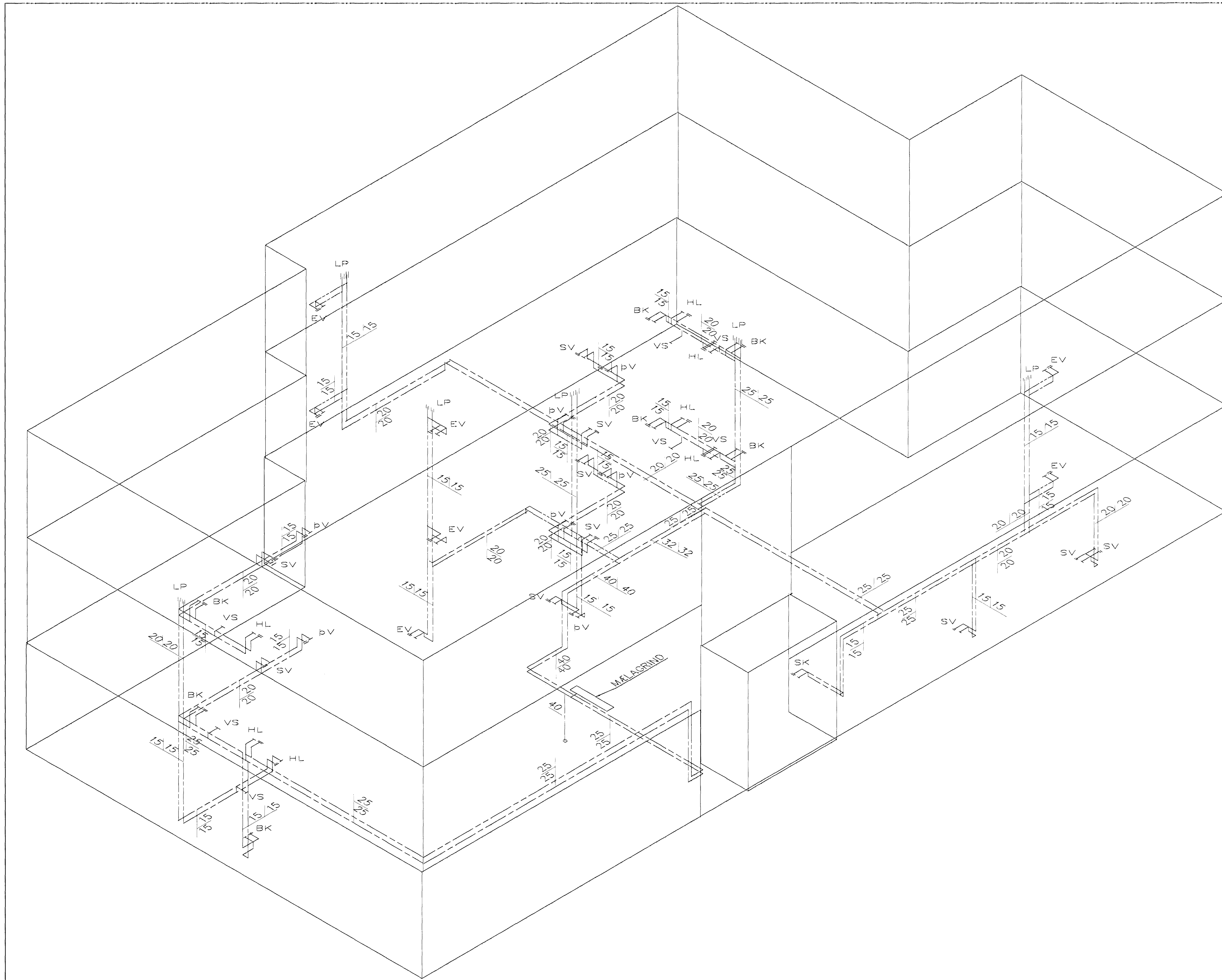
RÜMMYND VATSLAGNA 1:50
