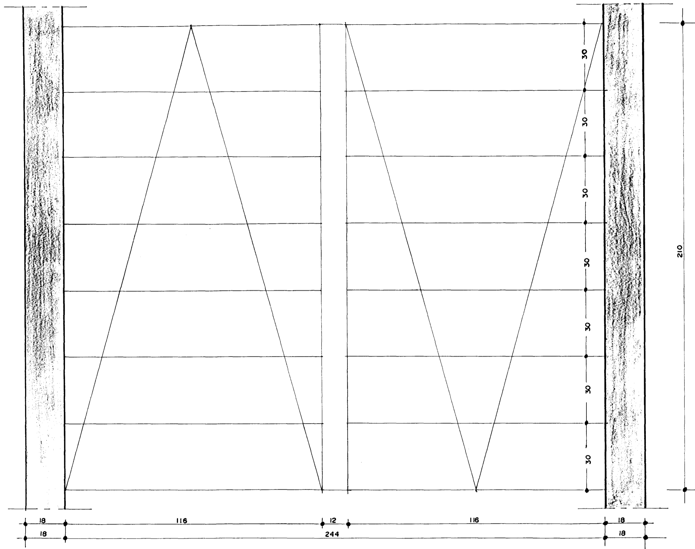
GRUNNMYND STIGI MKV. 1:10.
