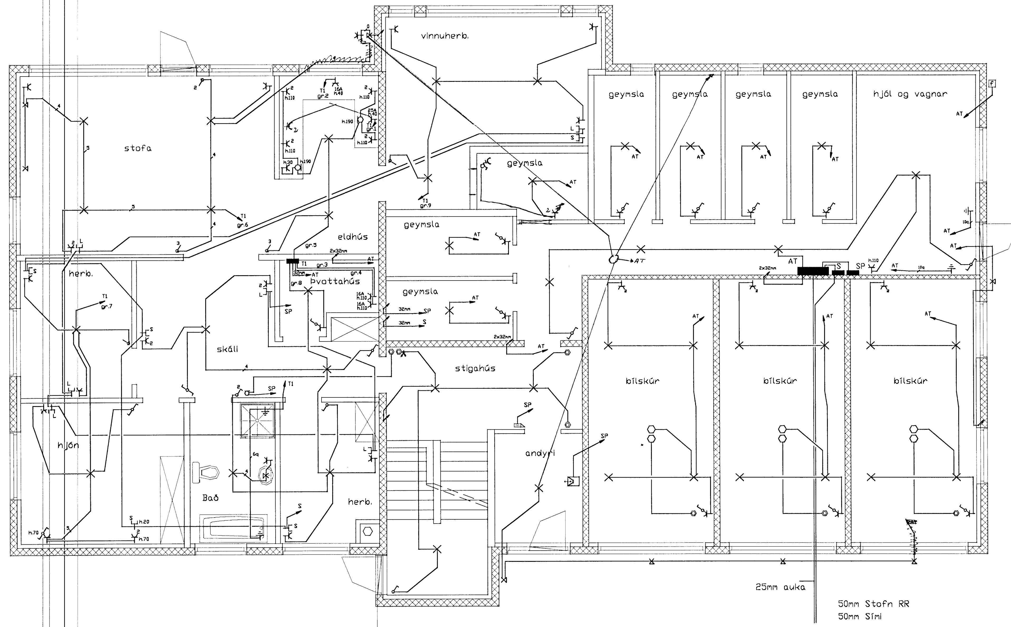
Grunnmynd 1:50
