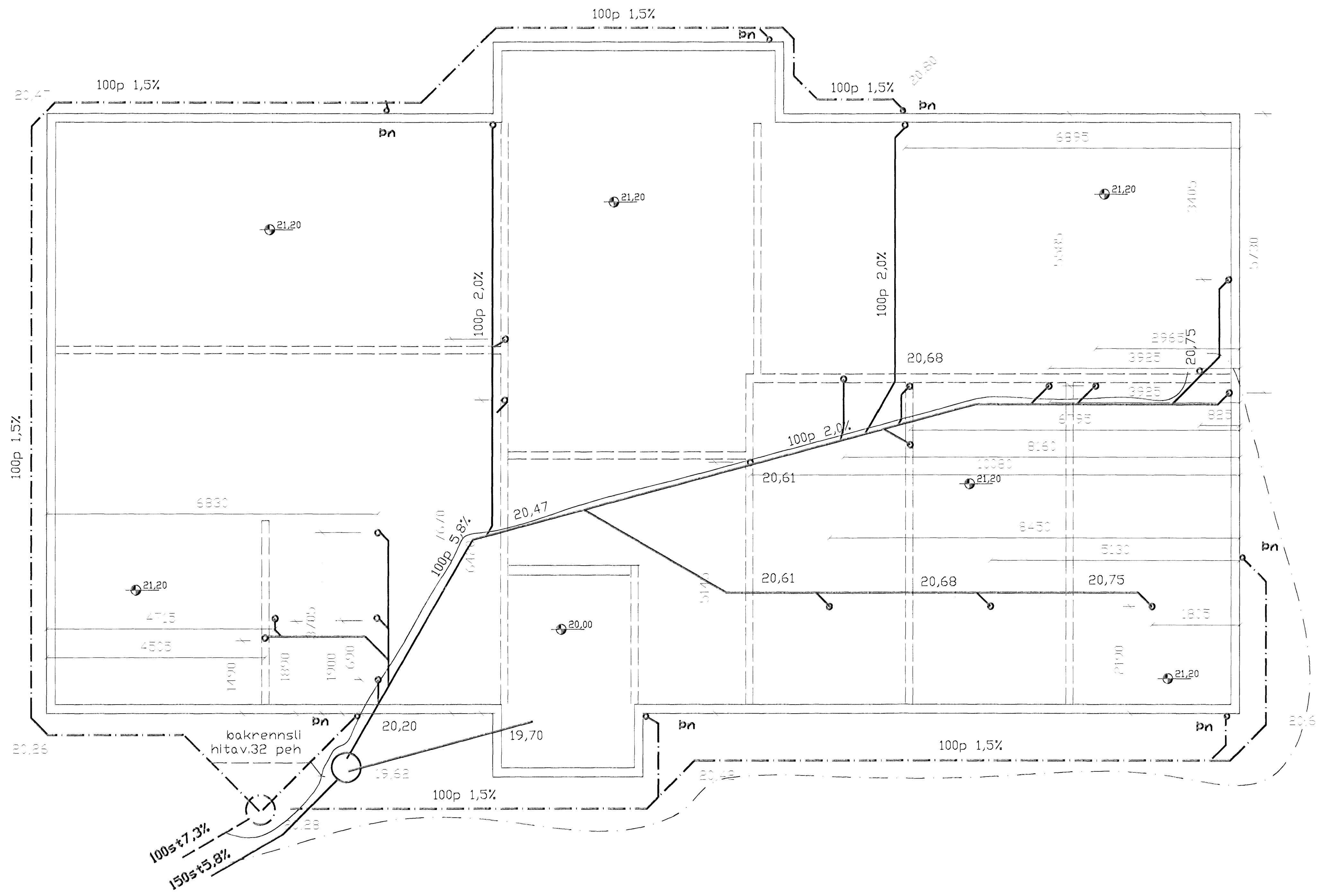
Grunnmynd 1/50
