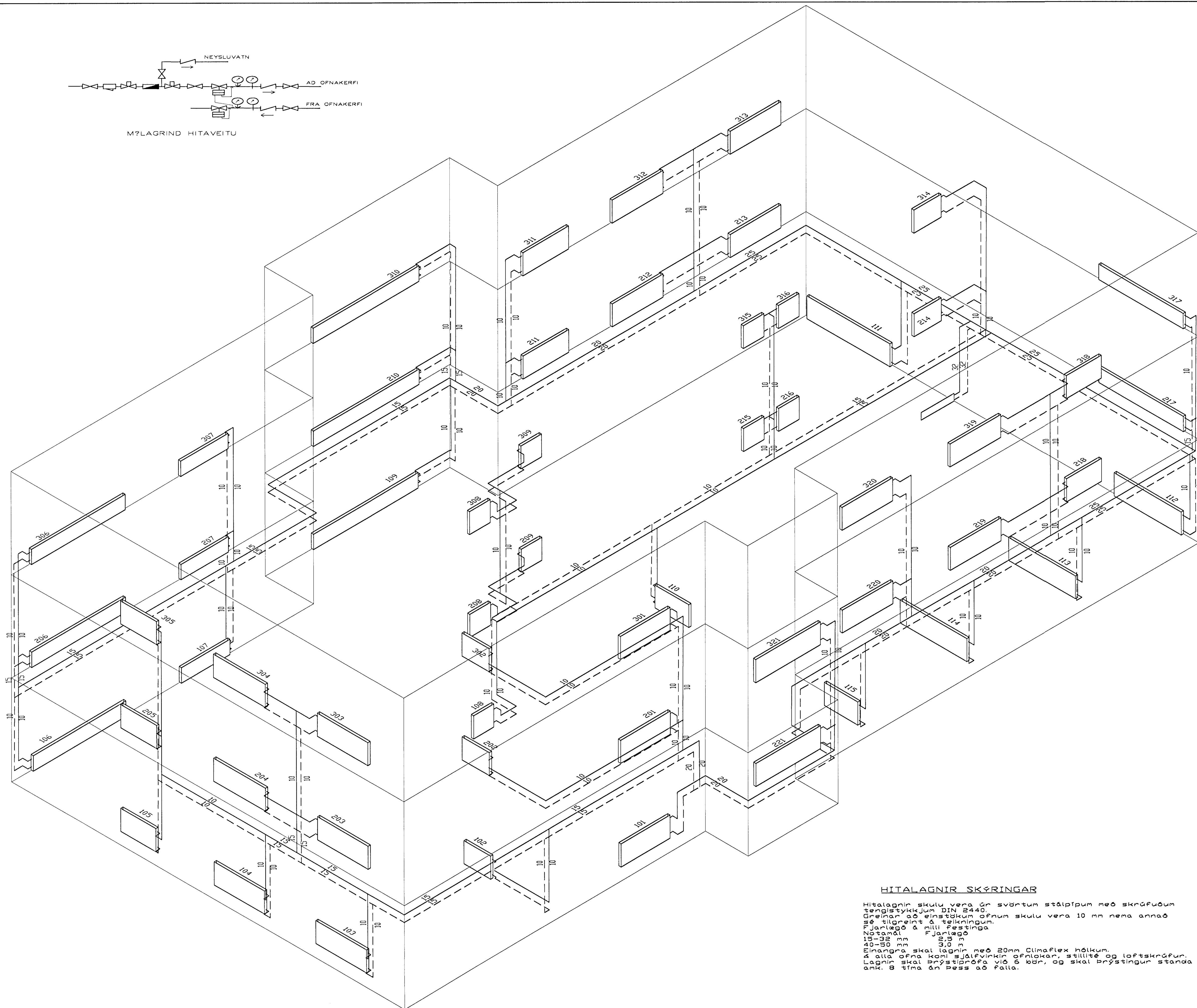
Hitalagnir, rúmynd, 1:50
