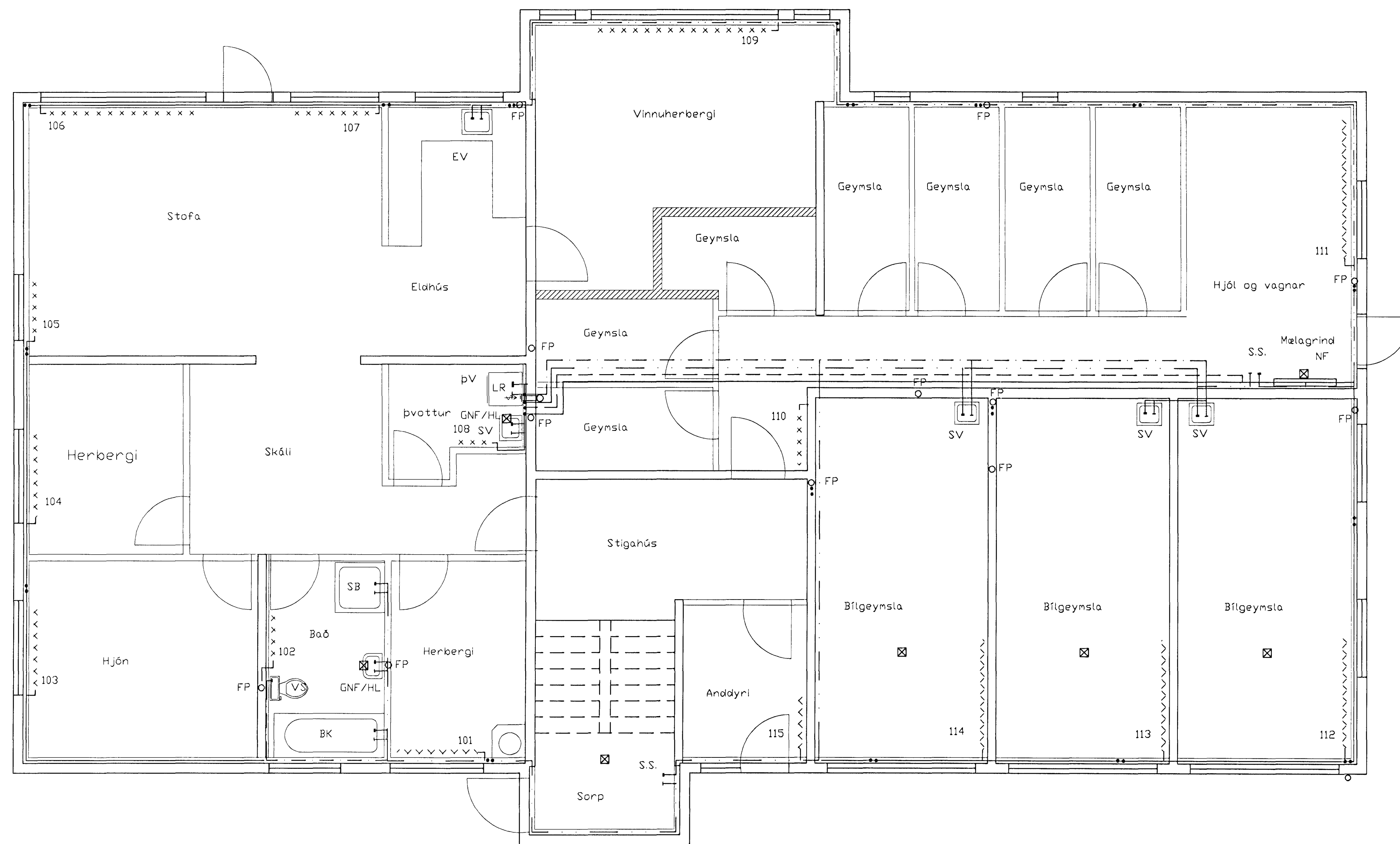
Lagnir 1. hæð, Grunnmynd, 1:50
